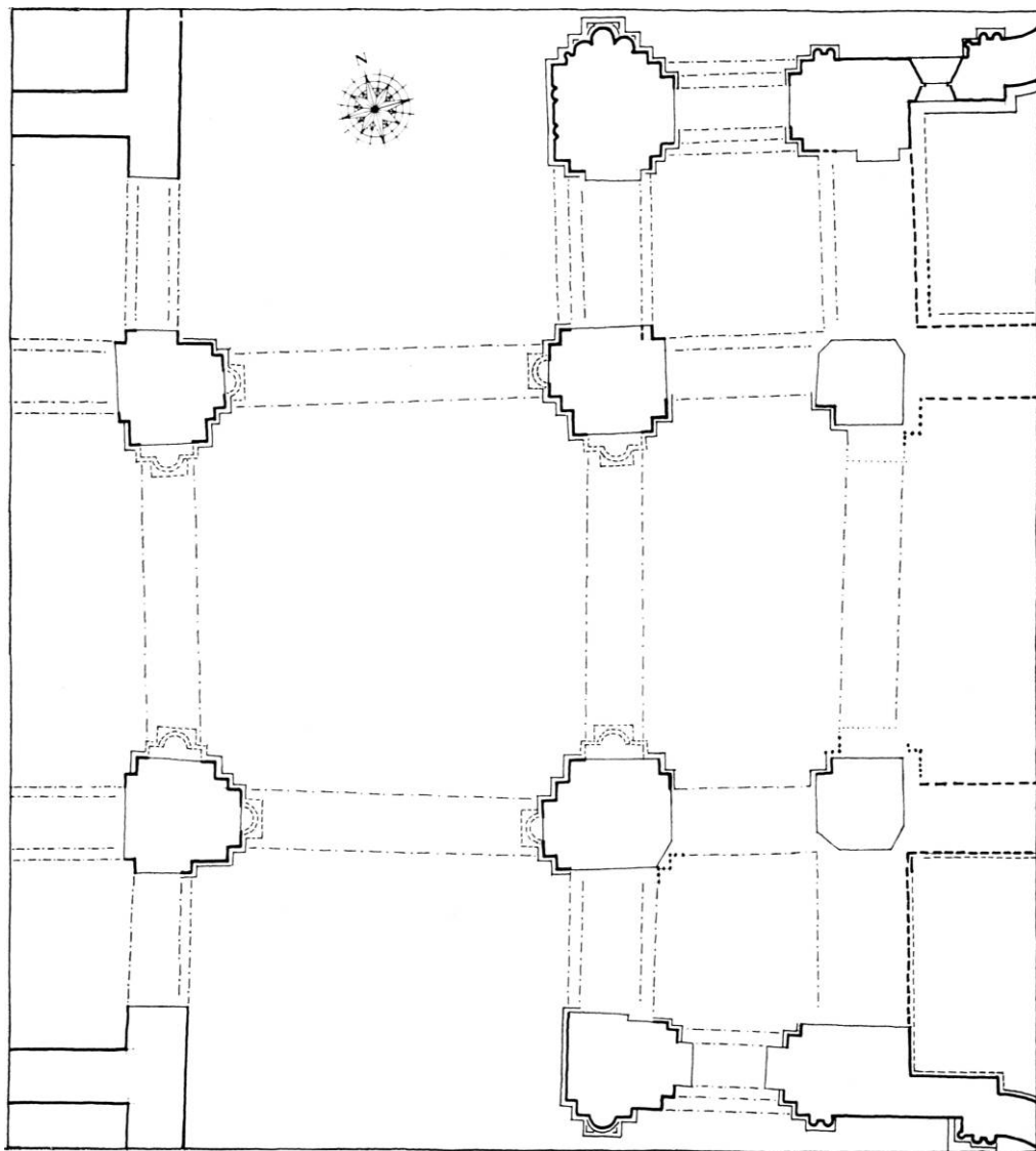
Fig. 40. Korsskæringen og nærmeste omgivelser, 1:200, med angivelse af oprindeligt murværk og sokkelforløb samt rekonstruktionsforslag og formodet størrelse af korkapellerne. KdeFL. (p. 144). — Crossing and area nearby, 1:200, with indication of original masonry and the course of the plinth, with suggestions for reconstruction and conjectured size of choir chapels.
