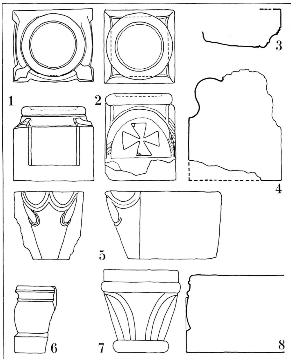
Fig. 173. Løstliggende granitblokke i og ved domkirken 1:10. 1 2 og 4 8 efter opmålinger af Jørgen Viemose (p. 343). 1. Jfr. fig. 190. 2. Jfr. fig. 175 og tegning af J. Ølsgaard i F. Beckett m.fl., Århus, København 1905, p. 125. 3. Karmsten, 79 cm lang, indmuret som overligger i åbningen mellem nordre kortårn og korets loft (p. 266)). 4. Jfr. fig. 31,1 og 58,5. 5. Jfr. p. 198 og fig. 95. KdeFL. - Granite blocks found in or by the cathedral 1:10. 3. Casing stone, 79 cm long, built in as lintel in the opening between the north choir tower and the loft of the choir.
