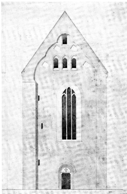
Fig. 162. Tværskibets sydgavl 1:300. Usigneret forslag i NM til istandsættelsen omkring 1880. — South side of transept. Unsigned suggestion for restoration c. 1880.
