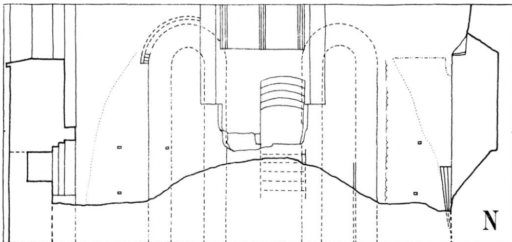
Fig. 85. Udsnit af indersiden af nordre korsarms mure ved det øverste galleri 1:100. KdeFL. Ø. Væggen på galleriets østside med spor af ældre hvælv og en rest af dettes ribbe; nedenunder: Plan af ribbelevnet 1:20. V. Væggen på galleriets vestside med omdannet vindue, jfr. fig. 87 (p. 209). N. Gavlvæggen med spor og rester af de oprindelige, rundbuede vinduer, jfr. fig. 118 (p. 150), for-tanding (p. 137), spor af ældre hvælv og tilhørende ribberest, jfr. fig. 86 (p. 205-06). Parts of the inner side of the walls of the north transept near the top gallery 1:100, and remains of vaulting rib 1:20.
