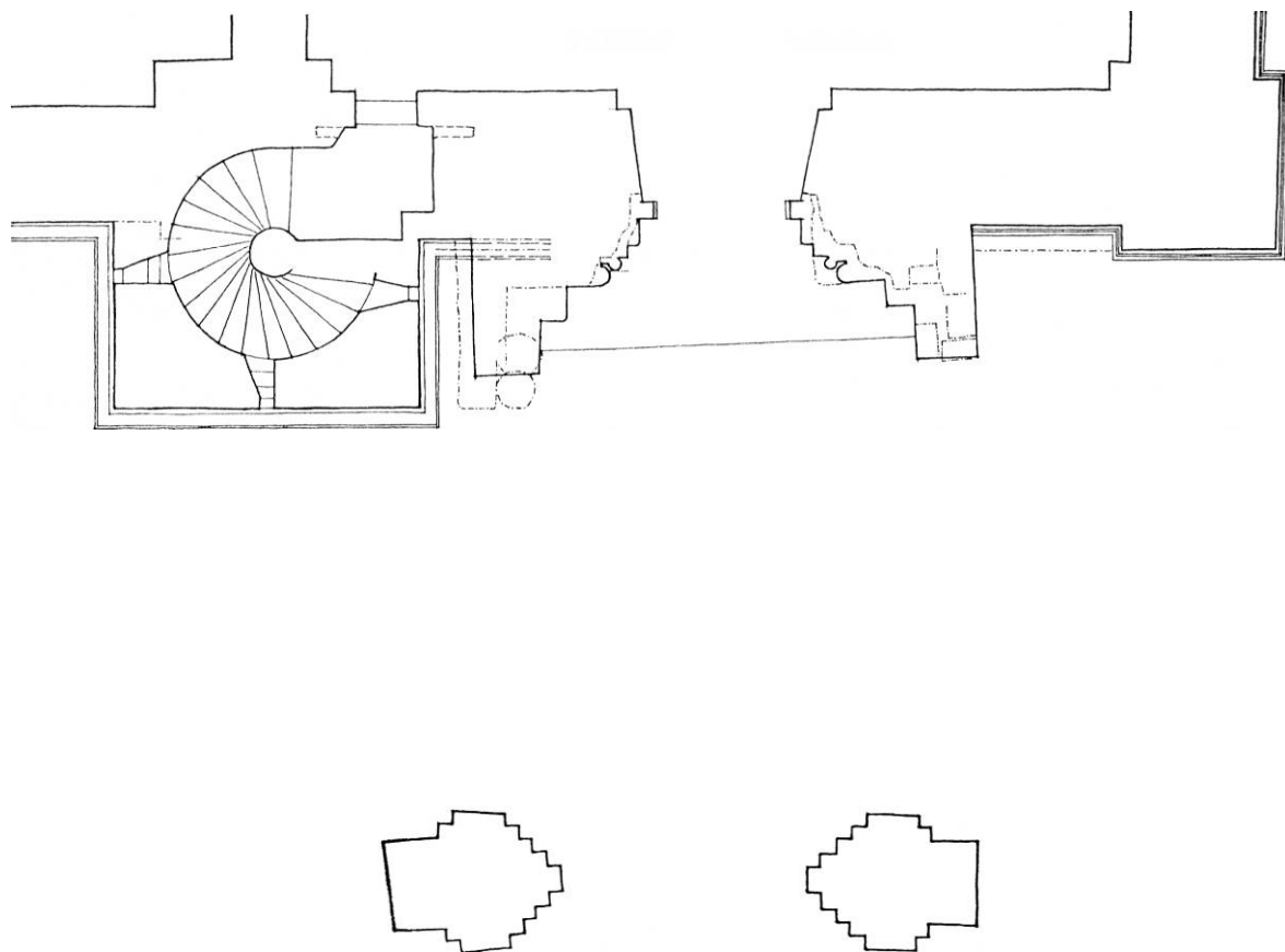
Fig. 54. Plan 1:100 af nordre korsarms nordgavl med angivelse af de rester og spor af fundering og sokkel, der registreredes ved portalens ombygning omkring 1880 (p. 157, jfr. fig. 53); tillige er indtegnet de piller fra broen til bispegården, som blev fremdraget 1926 (p. 104). Målt og tegnet af KdeFL 1968. — Plan scale 1:100 of north end of the north transept with indications of the remains and traces of foundation and plinth recorded during the rebuilding of the portal c. 1880; the piers from the bridge to the bishop's palace which were revealed in 1926 are also marked on the plan, cfr. fig. 96.
