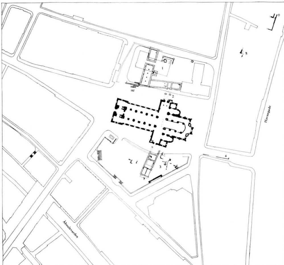
Fig. 20. Plan 1:2500 over området omkring Århus domkirke, tegnet af TF og KdeFL. Kortet viser kirken og levn af middelalderlige bygninger indtegnet på moderne gadeplan D 528 fra Stadsingeniøren i Århus.
