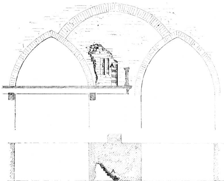
Fig. 80. Rester af det vestligste, oprindelige højkirkevindue fremhugget ved orgelpulpituret i langhusets nordside, som led i undersøgelserne forud for restaureringen i forrige århundrede 1:100. Tegning i NM af V. Th. Walther 1868 (p. 202). — Traces of the original west window in the nave on the north side, 1:100. Drawing by V. Th. Walther 1868
