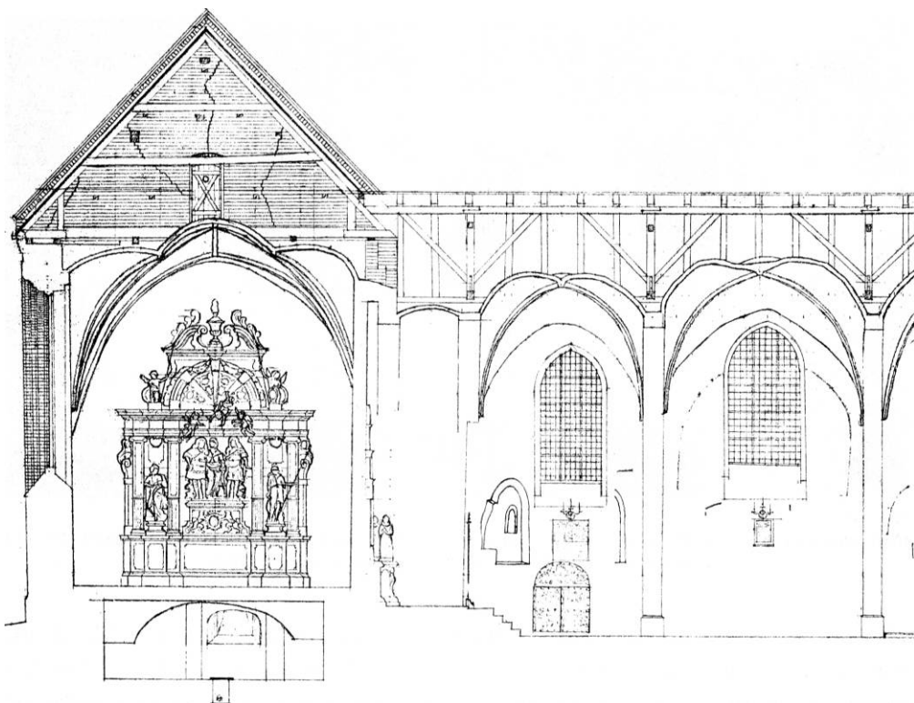
Fig. 92. Tværnit i nordre vestkapel med Marselis' epitafium og de to vestligste fag af nordre sideskib, set mod nord 1:200. Opmåling af Anton og Johannes Frederiksen 1907-15 (i domkirken) suppleret med den i 1920'rne fremhuggede niche i sideskibets vestligste fag, efter skitse af Jens Hougaard (p. 217). — Cross-section in the northern west chapel with Marselis's epitaph and part of the outer wall in the north side aisle 1:200.
