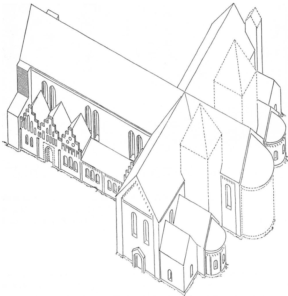
Fig. 88. Axonometrisk rekonstruktionsskitse af domkirkens ydre set fra sydøst for påbegyndelsen af 1400-tallets ombygninger, 1 : 600, KdeFL. Ligesom for fig. 35 gælder det, at der savnes grundlag for bestemmelse af højcorets oprindelige ostafslutning (p. 139); tillige er det usikkert, om de på tegningen punkterede tårne over de indre østkapeller nogensinde nåede højere end tværskibets tagfod (p. 176—79). Hvad angår søndre sideskibs ombygning, skal skråprojektionerne illustrere, at forandringerne formentlig blev foretaget fag for fag (p. 215—16), men det skal understreges, at udformningens enkeltheder kendes ikke. — Axonometric sketch for the reconstruction of the exterior of the cathedral seen from the southeast before the rebuilding in the 15th century.
