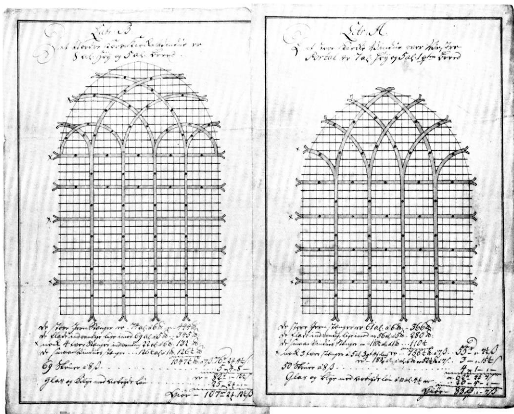
Fig. 151. H.Næss: To forslag til vinduer ca. 1772, dels i nordre korsarm, dels i vestfronten. Landsarkivet, Viborg. — H.Næss: Two drafts for windows c. 1772. The archives, Viborg.
