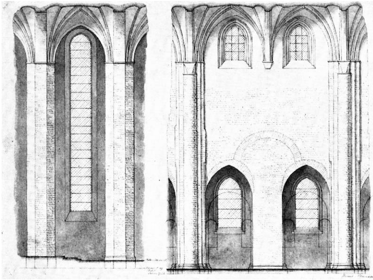
Fig. 81. Udsnit af søndre pillerække i koret samt et fag i langhuset med indtegnet rekonstruktionsforslag, 1:300. Laveret tegning af Heinrich Hansen 1855 i NM. — Section of row of piers in the south side of the choir, together with a bay in the nave with suggestions for reconstruction, 1:300. Drawing in colour wash by Heinrich Hansen 1855.
