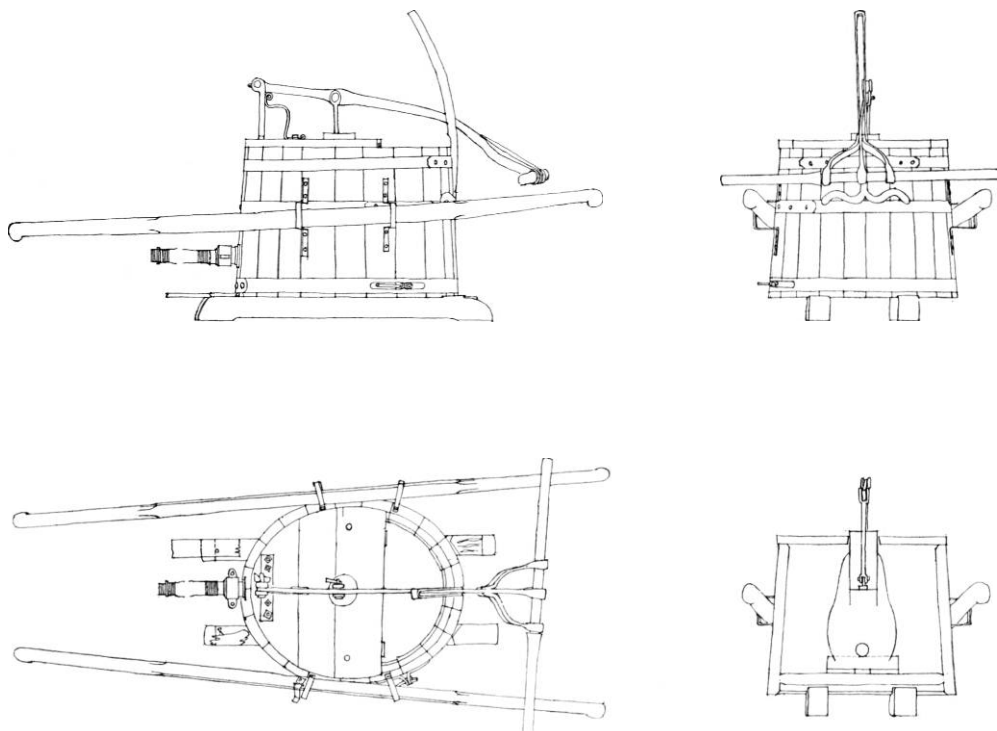
Fig.172. Brandsprøjte på domkirkens loft, ca. 1:25. Målt og tegnet 1968 af Jens Hougaard og H.C.Wessing. Arkitektskolen i Århus. — Fire-pump in the loft of the cathedral, c. 1:25.
