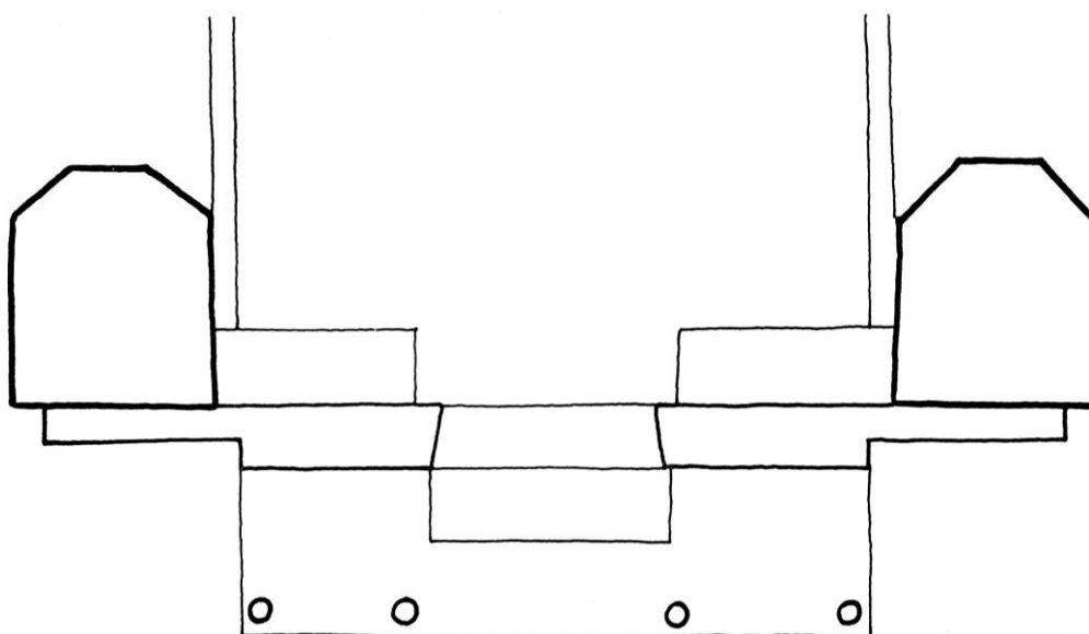
Fig. 136. Østre korsskæringspiller og lektoriet, plan 1 :100, tegnet af KdeFL efter Cramers gravkort 1745, jfr. fig. 150 (p. 276). East piers of the crossing and the lectorium 1:100, sketched after Cramer's map 1745, cf. fig. 150.
