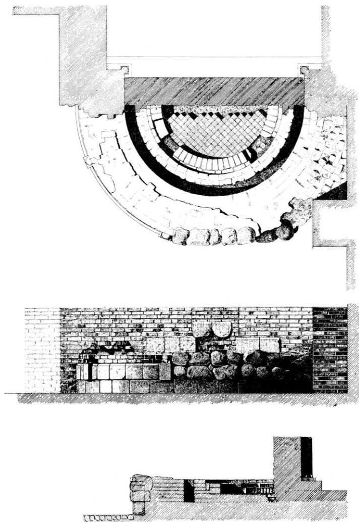
Fig. 159. Rester af fundament og sokkel på søndre apsiskapel, ca. 1:100 (p. 174 og 323). Opmåling i NM af S.F. Kühnel 1880. — Remains of foundation and plinth in the south apse chapel c. 1:100, survey 1880.
