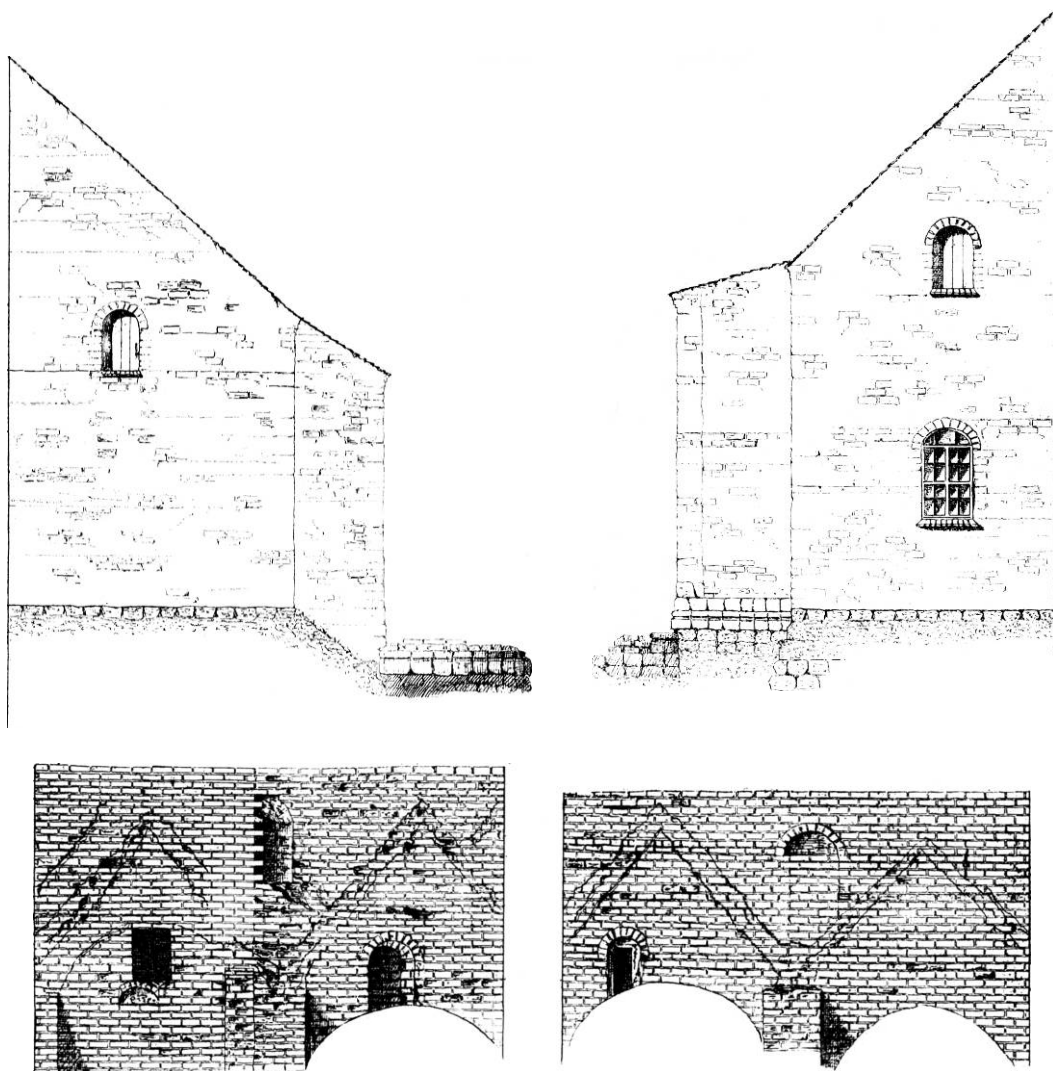
Fig. 160. Østkapellerne 1:200. Opmåling i NM, udført før bygningernes restaurering omkring 1880. — East chapels 1: 200. Survey made before the restoration of the buildings c. 1880.
