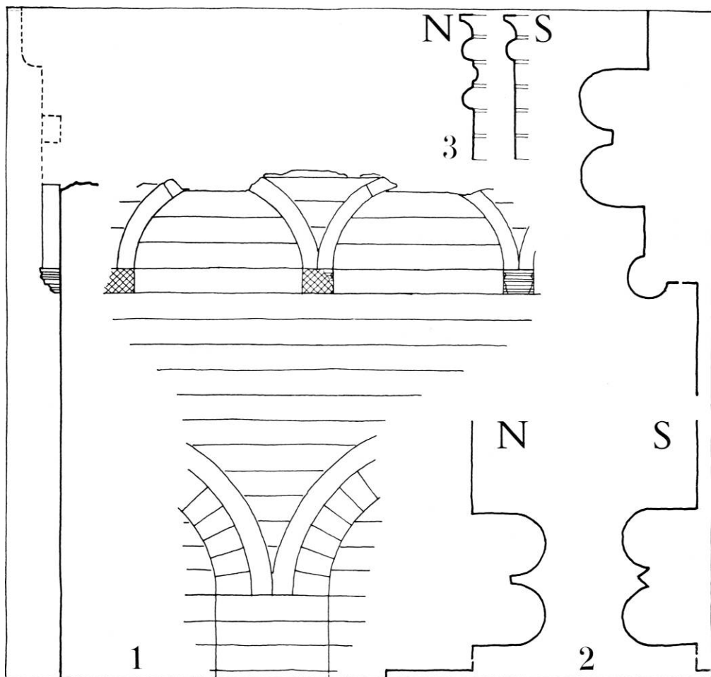
Fig 66. Enkeltheder fra ostafsnittet 1:20. 1. †Façadeparti på nordre apsis (p. 181), KdeFL. 2. Væg-piller i søndre apsiskapel (p. 172). 3. Kragbånd (p. 172 og 183). 2 og 3 tegnet af KdeFL efter C. M. Smidt. — Details from the east section 1:20. 1. Part of the façade of the north apse. 2. Pilasters in the south apsidal chapel. 3. String courses.
