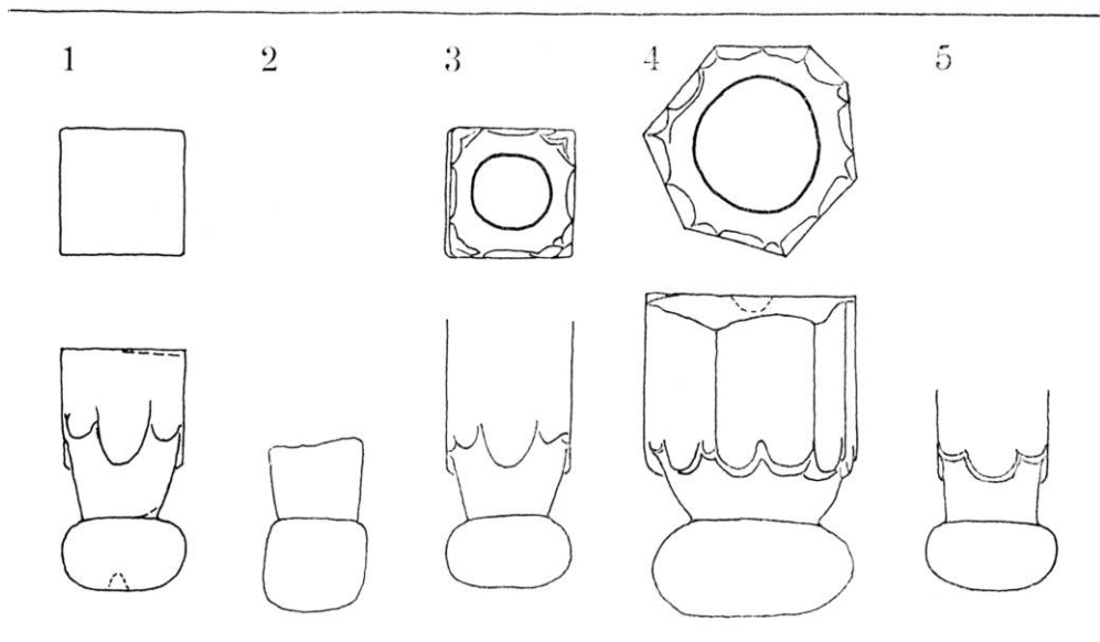
Fig. 68. Hvælvingslutsten af granit, 1:10, KdeFL. 1. Om Klostermuseum, fra Borgergade 34, Skanderborg. 2. Stiftsmuseet, Viborg (museums nr. 6609), efter Levin Nielsen 1966. 3. Nordlige afvisersten ved porten Mejlgade 74, Århus. 4. Vejlbj kirkegård, Århus (jfr. fig. 181). 5. Apsis, Grøn-bæk kirke, efter C. M. Smidt 1924 (p. 185). — Keystones from vaults 1:10. 1. Om Abbey Museum, from Borgergade 34, Skanderborg. 2. The Museum, Viborg (museum no. 6609), after Levin Nielsen 1966. 3. North stone post at the gateway Mejlgade 74, Århus. 4. Vejlbj churchyard, Århus. (cfr. fig. 181) 5. Apse, Grøn-bæk church, after C. M. Smidt 1924.
