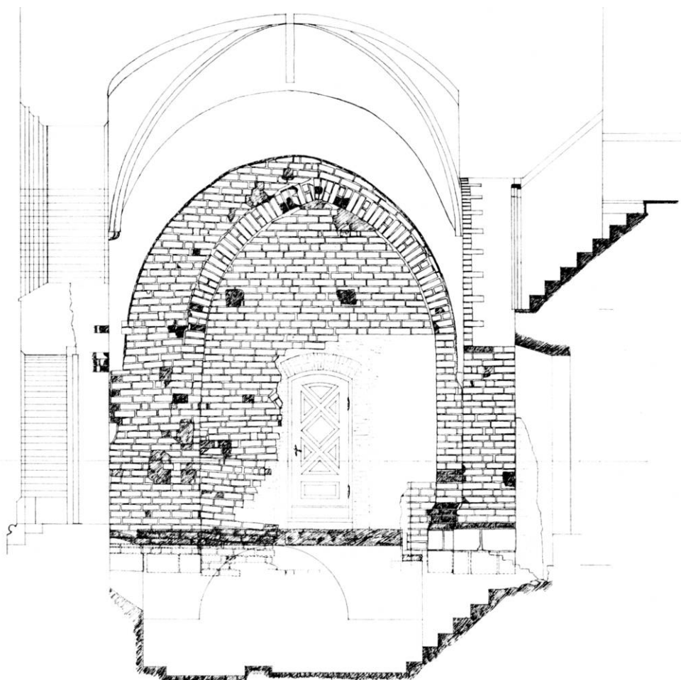
Fig. 74. Nordligste ostkapels sydvæg 1:80 efter opmåling af Johannes Frederiksen 1908, forud for rummets istandsættelse (p. 327). På tegningen ses sporet efter kapellets oprindelige overhvælving (p. 188), den formentlig oprindeligt åbne arkade ind til nordre apsiskapel (p. 187) samt rester af stikket og vestre hjørne af åbning i denne arkades tilmuring (p. 187). Af nyere indretninger bemærkes i øst-væggen vindue og dør, således som de blev udformet ved restaureringen omkring 1880 (p. 323); under det hævede gulv er Lindenows gravkælder med opgang og gennembrydning af muren til tværskibet, samt herover den sekundære, nu fjernede trappe til nedre galleri i nordre korsarm (p. 287). — The south wall of the northernmost of the east chapels as in 1908 before the restoration. 1: 80.
