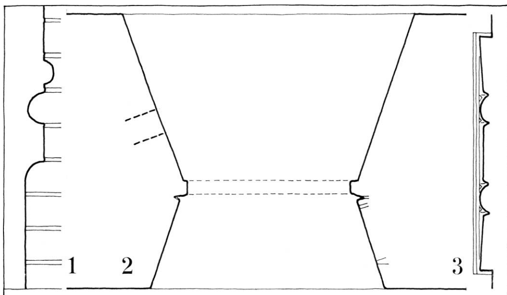
Fig. 46. Detaljer fra tværskibet: 1. Sokkel på pillen på nordre korsarms vestvæg 1:10 (p. 206). 2. Søndre korsarms nordligste vindue i vestvæggen 1:20 (p. 150). 3. Søndre halvøjlepille i nordre korsarm 1:40. KdeFL. (p. 142). — Details from the transept. 1. Pier plinth at the west wall of the north transept 1:10. 2. Window furthest to the north in the west wall of the south transept 1:20. 3. South pilaster in the north transept 1:40.
