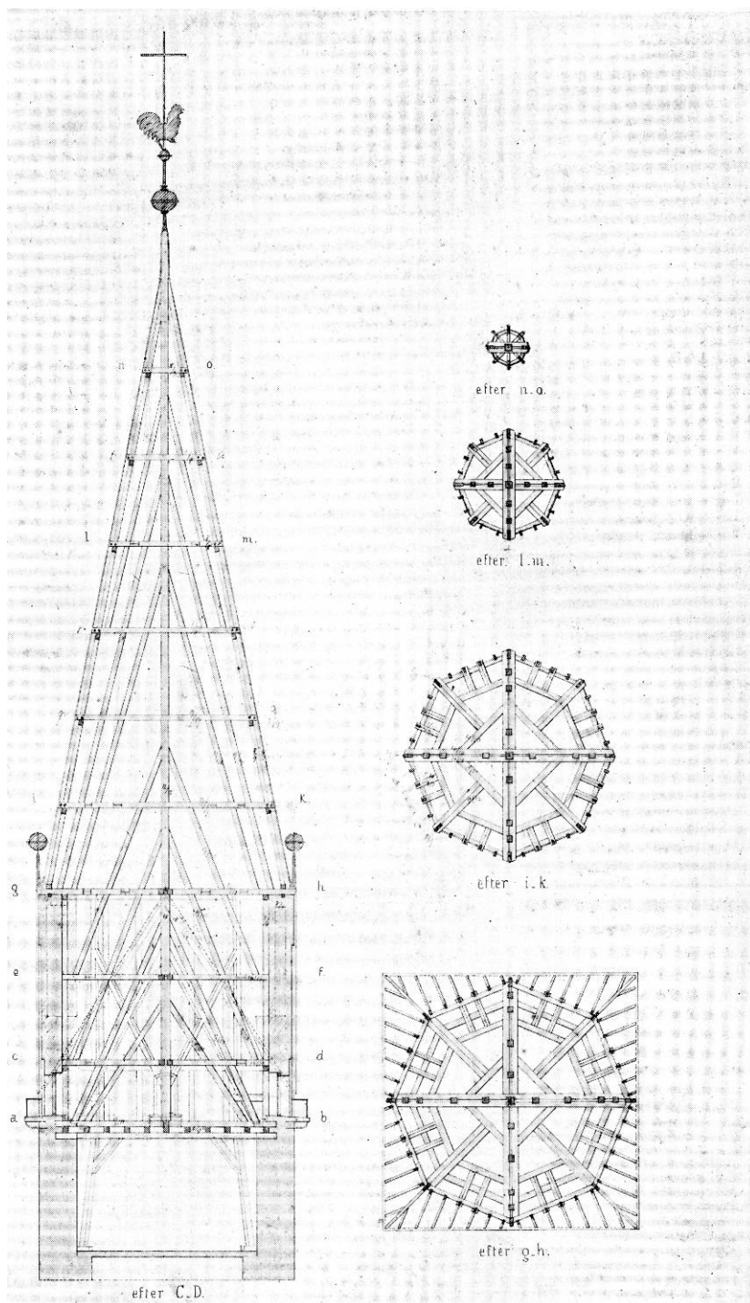
Fig. 163. Udsnit af V. Th. Walthers tegning 1876 til spir på vesttårnet. I domkirken. V. Th. Walther's drawing 1876 for a spire on the west tower.
