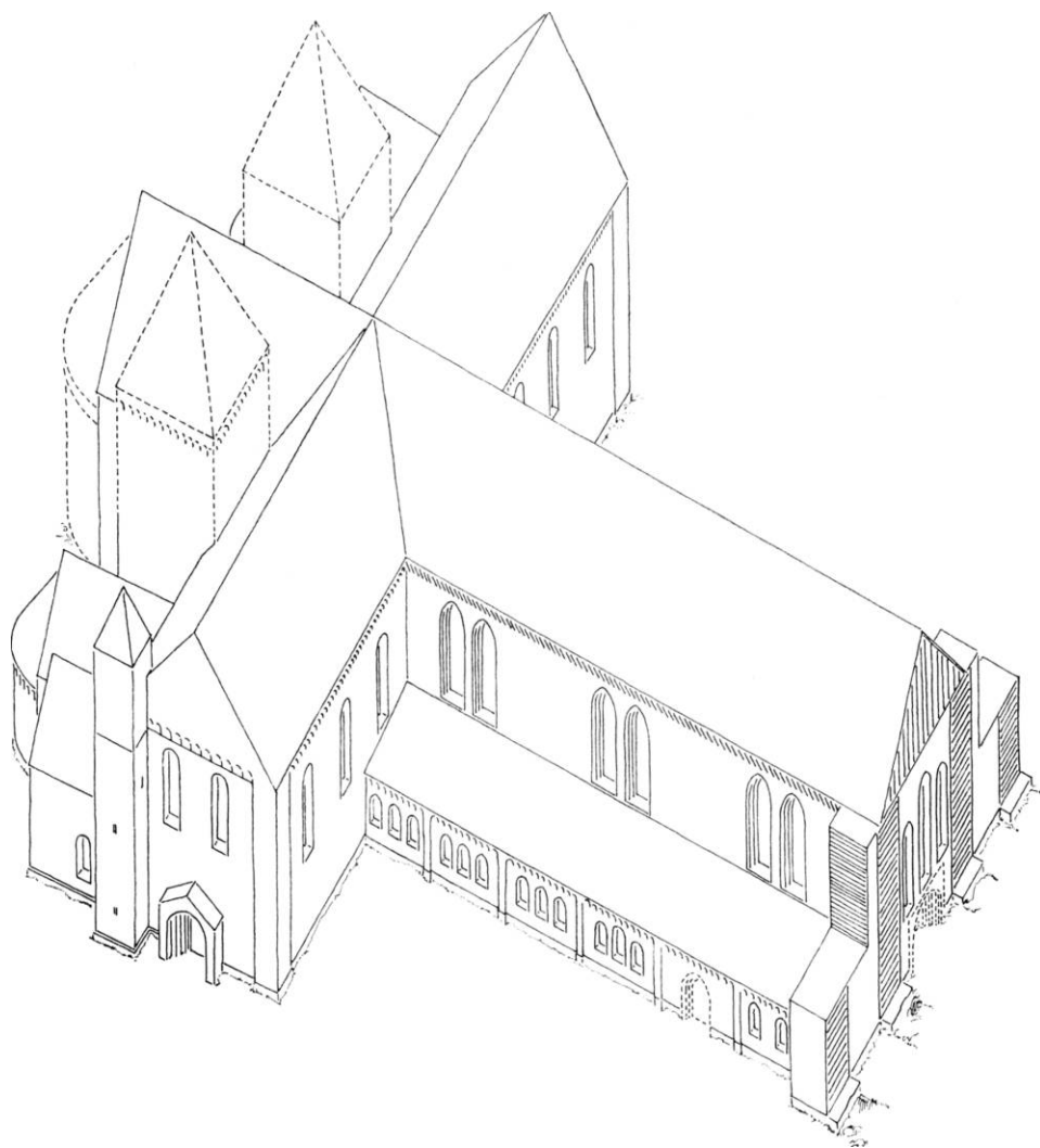
Fig. 35. Axonometrisk rekonstruktionsskitse af domkirkens ydre, set fra nordvest efter afslutningen af langhusets opførelse 1:600. KdeFL. Udformningen af højkorets ostafslutning er usikker (p. 139), det samme gælder for de mulige kortårne (p. 176). Enkeltheder som friser og langhusets portaler er hypotetiske; vestgavlens fortandinger markerer det afbrudte byggeri (p. 198). — Axonometric sketch for the reconstruction of the exterior of the cathedral, seen from the northwest after the building of the nave had been completed.
