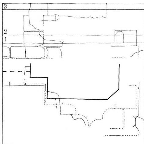
Fig. 177. Sokkelforholdene på sydsiden under den næstvestligste pille i korets nordside; opstalt og plan 1:60, KdeFL 1969. 1. Formentlig oprindeligt gulvniveau. 2. Gulvhøjde i nuværende koromgang. 3. Gulvniveau i højkoret (p. 139). — Position of plinths to the south under the pier second from the west at the north side of the choir 1:60. 7. Possibly the original floor level. 2. Floor level in the present ambulatory. 3. Floor level in the choir.
