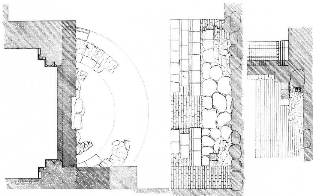
Fig. 69. Rester af fundament og sokkel på nordre apsis kapel, ca. 1:100; tillige ses lukkemuren, der opsattes efter apsidens nedbrydning. Opmåling i NM af S. F. Kiihnel 1880 (p. 180). — Remains of foundation and plinth of the north apse chapel c. 1:100 Survey by S. F. Kiihnel 1880.
