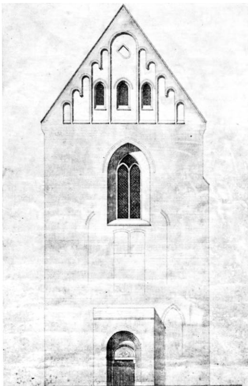
Fig. 161. Tværskibets nordgavl 1:300. Usigneret forslag i NM til istandsættelsen omkring 1880. — North side of the transept. Unsigned suggestion for restoration c. 1880.
