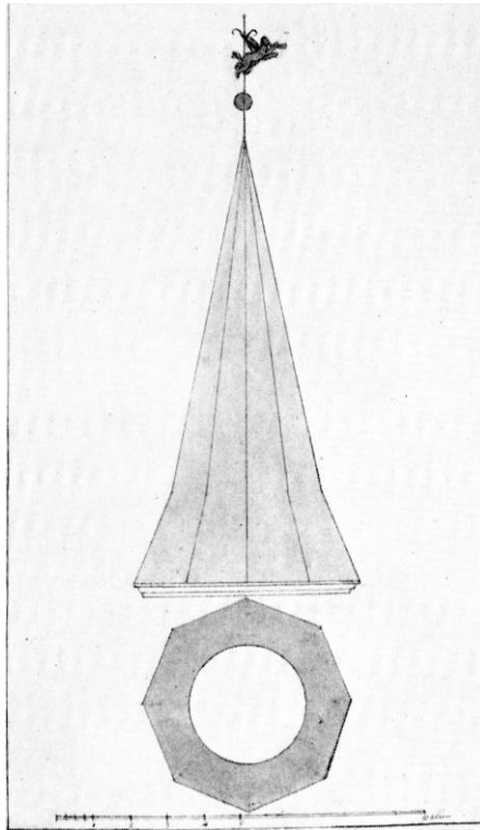
Fig. 153. Forslag til kortårnespir 1822, vist af B.Bonnesen. Landsarkivet, Viborg — Suggestion for spire on the choir towers 1822. The archives, Viborg.
