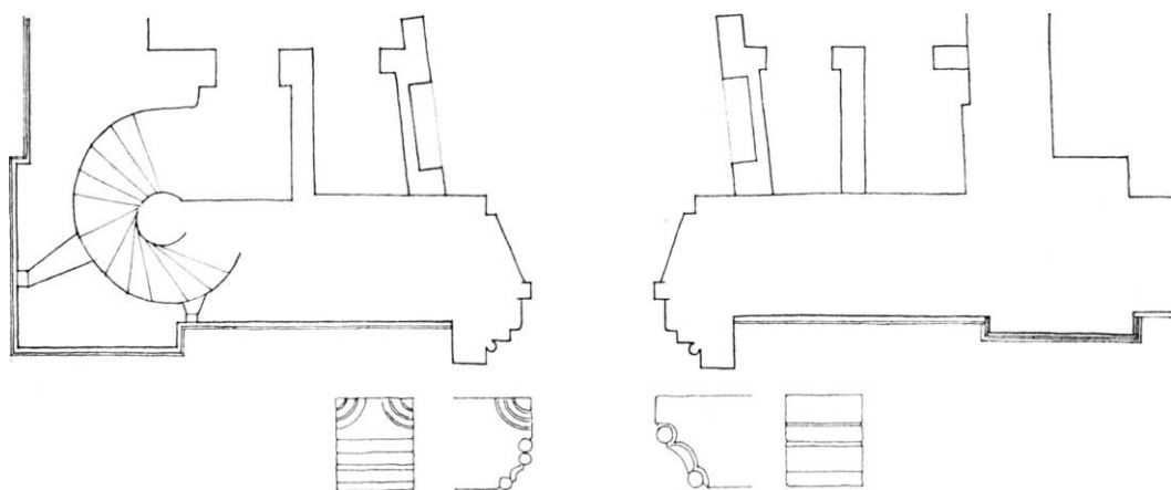
Fig. 49. Søndre korsarms gavl, plan 1:100, KdeFL 1965, og portalens kragsten 1:20, målt af Jørgen Viemose (p. 153). — The south end of the south transept 1:100 and the corbels of the ported 1:20.
