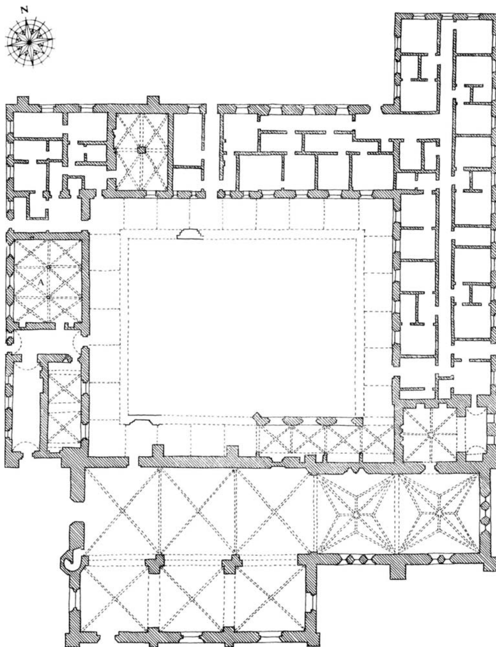
Fig. 4. Vor Frue kirke og Århus hospital, kaldet Vor Frue kloster. Grundplan 1:400 af kompleksets rumindretning 1976, jfr. p. 1013, fig. 5. Tegnet af KdeFL på grundlag af p. 1043, fig. 30 (kirken), tegninger af Aksel Skov 1950 og 1955 samt af Jørgen Malling og Jens Vilhelmsen 1975 (fløjene), C. M. Smidt 1905 og C. G. Schultz 1957 (korsgangen). Nuværende hospitalskirkesal mærket A. Ground plan 1:400 of the complex 1076, cf. p. 1013, fig. 5. The present hospital chapel marked A.
