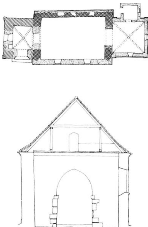
Fig. 3. Skejby. Plan 1:300, målt 1966 og tegnet af KdeFL. — Groundplan 1:300. Fig. 4. Tværsnit i skibet, set mod øst, 1:150. Målt 1966 og tegnet af KdeFL. — Crosssection in the nave, looking east, 1:150.
