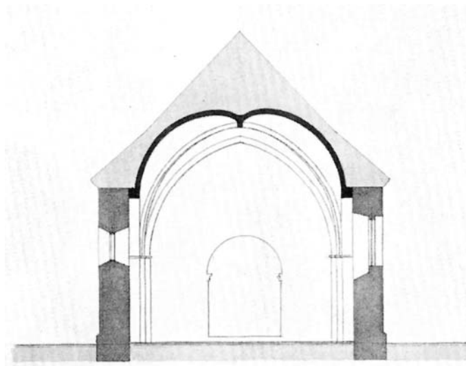
Fig. 3. Åby. Den 1872 nedrevne kirke, tværnsnit i skibet 1:150, set mod øst. Opmåling 1872 ved V. Th. Walther. (NM). — The demolished church. Cross-section in the nave looking east, 1872, 1:150.
