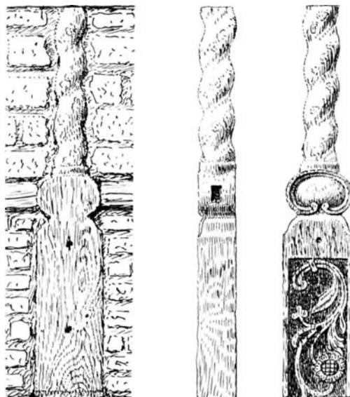
Fig. 23. Brabrand. *Pulpitursøjle(?) indmuret i gården »Engkjær«, nu Truegården, Frilandsmuseet. Tegning 1925, 1:20, af Søren Knudsen (p. 1537). Column of pew gallery(?) re-used in a farm-house, now in the »Frilandsmuseum« at Sorgenfri.
