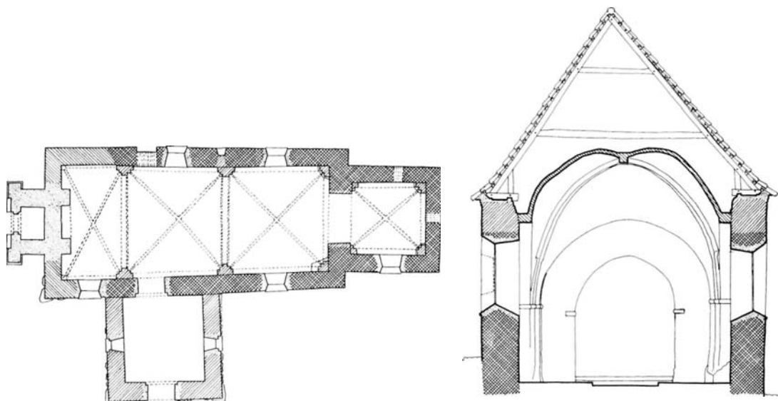
Fig. 2. Sdr. Årslev. Plan 1:300, målt af TF og KdeFL 1969. - Ground-plan 1:300. Fig. 3. Sdr. Årslev. Snit 1:150, målt af TF og KdeFL 1969. - Cross-section 1:150.
