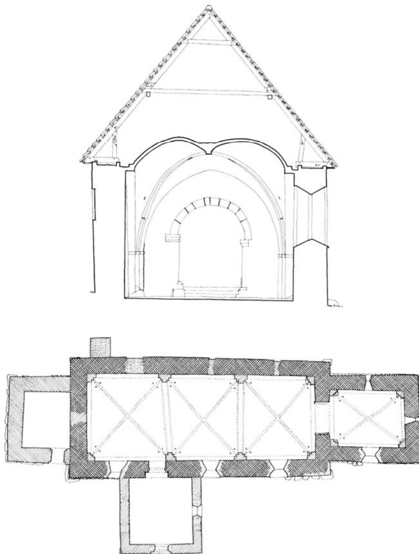
Fig. 3. Tilst. Tværsnit 1:150. Målt og tegnet af TF og KdeFL 1969. — Cross-section 1:150. Fig. 4. Tilst. Plan 1:300. Målt og tegnet af TF og KdeFL 1969. — Ground-plan 1:300.
