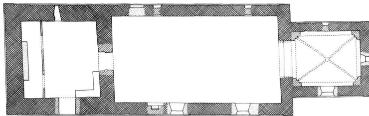
Fig. 2-3. Plan 1:300 og tværsnit 1:150. Målt af KdeFL og HJ 1967, tegnet af Flemming Beyer 1980. - Ground-plan 1:300 and cross-section of the nave 1:150.
