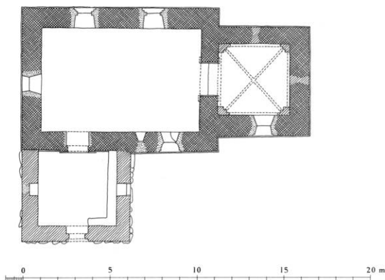
Fig.2-3. Plan 1:300 og tværsnit af skib 1:150. Målt af HJ og KdeFL 1966, tegnet af Flemming Beyer 1981. - Ground-plan 1:300 and cross section of nave 1:150.
