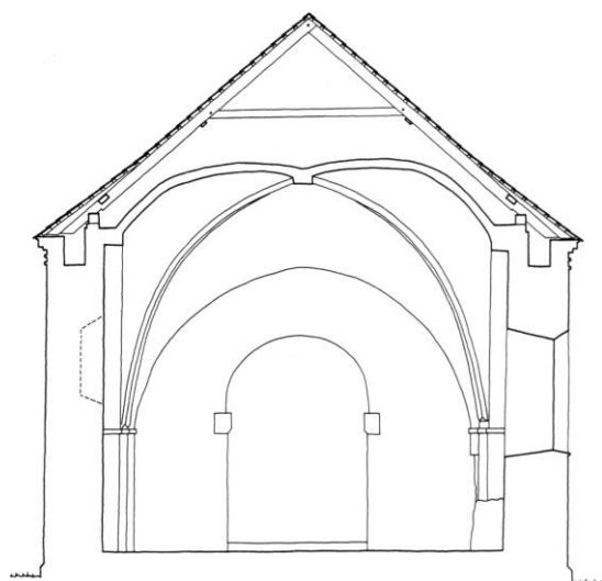
Fig. 6. Tværnsnit af skib 1:150. Målt af Jens Hougaard og Jørgen Viemose 1970, tegnet af Flemming Beyer 1981. - Cross-section of nave, 1:150.
