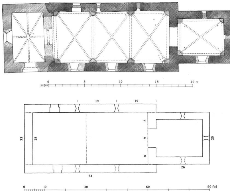
Fig. 2. Plan 1:300. Målt af J.Hougaard og J.Viemose 1970, tegnet af Fl. Beyer 1981. - Ground-plan 1:300.
