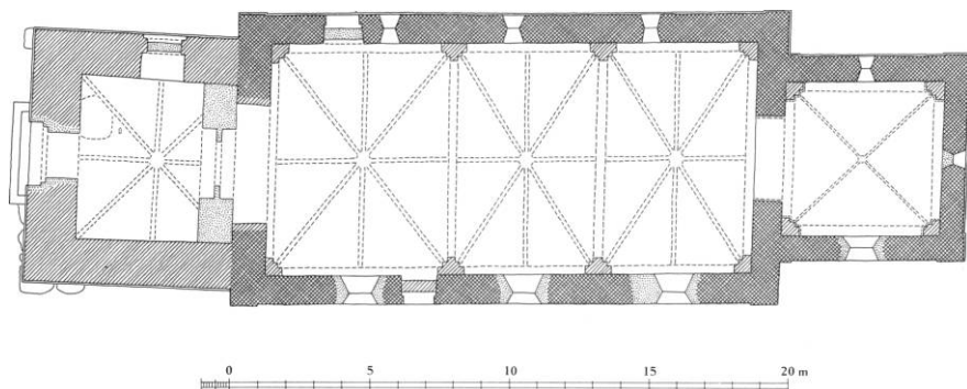
Fig.2-3. Plan 1:300 og tværsnit af skib 1:150. Målt af Jens Hougaard og Jørgen Viemose 1970, tegnet af Flemming Beyer 1981. - Ground-plan 1:300 and cross section of nave 1:150.
