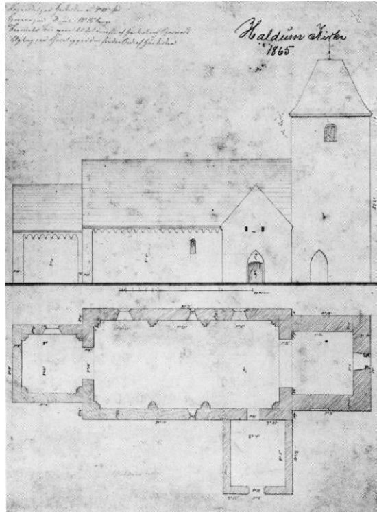
Fig. 4. Plan og opstalt 1865, før ombygningen. Sandsynligvis tegnet af Christen Kiilsgaard. LA Vib. - Plan and elevation 1865, before renovation.
