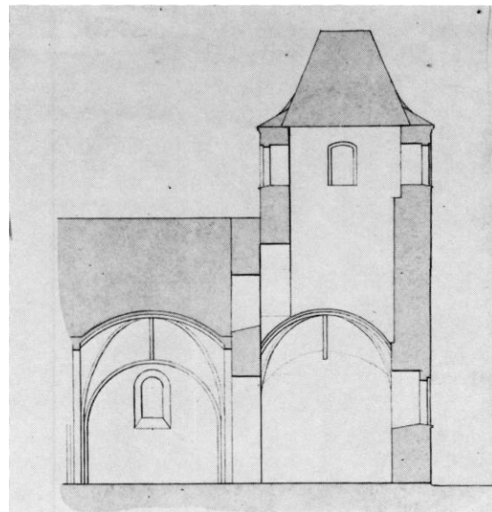
Fig. 5. Snit gennem skib og tårn. Formodentlig tegnet af Christen Kiilsgaard 1865. LA Vib. - Sectional view of nave and tower.
