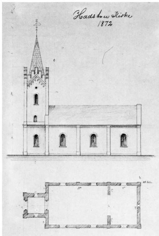
Fig. 4. Forslag til ny kirke, tegnet af Christen Kiilsgaard 1872. - Design for new church 1872.
