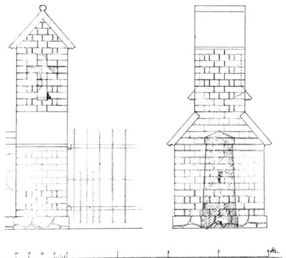
Fig. 3. Forslag til murede portpiller, formentlig tegnet af Christen Kiilsgaard (s. 1848). - Design for gateports, presumably drawn by Christen Kiilsgaard.
