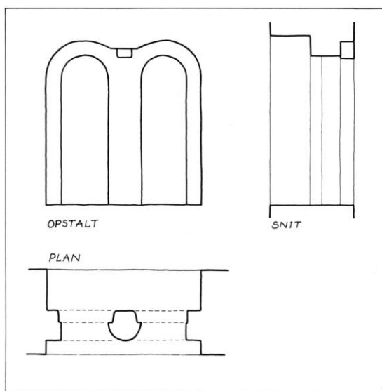
Fig. 5. Tårnets østre glamlul (s. 2092), 1:50. Målt af J. Hougård og J. Viemose 1970, tegnet af Marianne Nielsen 1982. - East belfry light of the tower.
