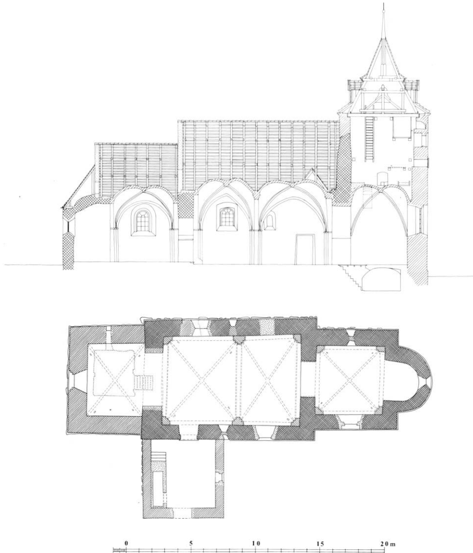
Fig. 2. Længdesnit 1:300, set fra nord. Målt og tegnet af Børge Sander Sørensen, Torsten Hinge, Erik Rasmussen og Vagn Kjeld Andersen, Arkitektskolen i Århus 1973. - Longitudinal section 1:300.
