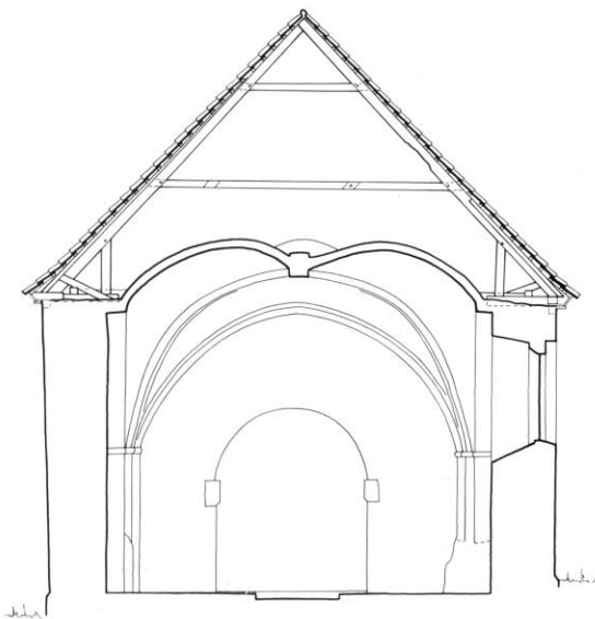
Fig. 5. Tværsnit gennem skib 1:150, målt af Jens Hougård og Jørgen Viemose 1971, tegnet af Marianne Nielsen 1983. - Cross-section of the nave 1:150.
