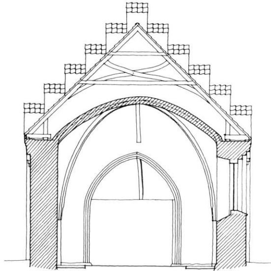
Fig. 4. Tværnsnit gennem langhuskorets østre fag set mod øst, 1:150. Målt og tegnet af Kristian Agger, Ernst Kallesøe og O. Østergård, Arkitektskolen i Århus. - Cross-section of chancel 1:150.
