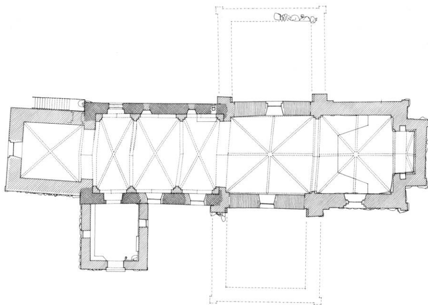
Fig. 2. Længdesnit 1:300, målt og tegnet af Kristian Agger, Ernst Kallesøe og O. Østergård, Arkitektskolen i Århus 1970-71. - Longitudinal section 1:300.
