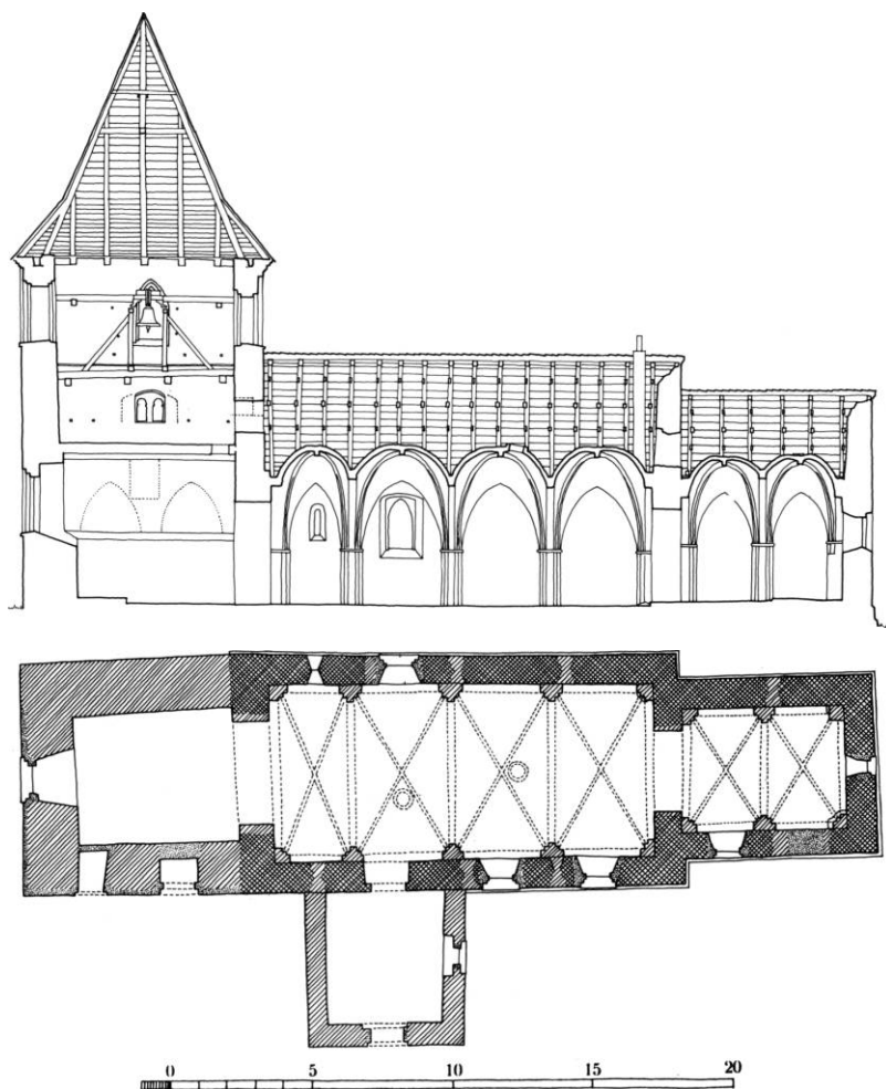
Fig. 6-7. Plan og længdesnit 1:300. Målt af Gert Bech-Nielsen, Ebbe Gitz-Johansen og Alfred Hansen 1968, tegnet med enkelte suppleringer af KdeFL 1983. - Plan and longitudinal section 1:300.
