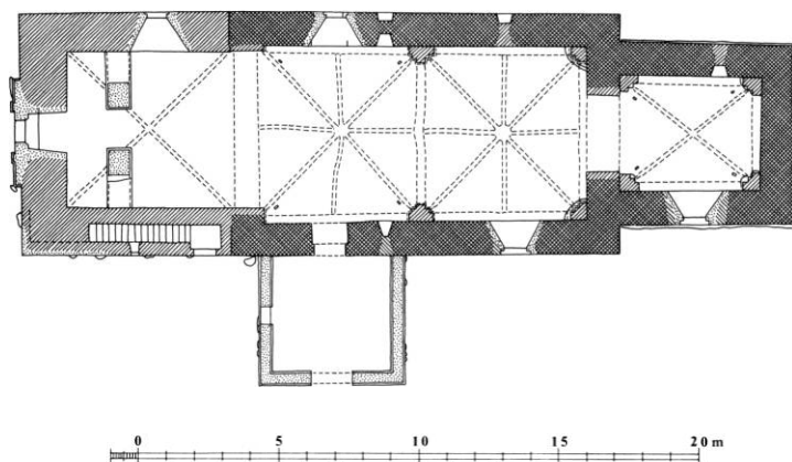
Fig.2. Plan 1:300. Målt af Jens Hougård og Jørgen Viemose 1970, tegnet af Marianne Nielsen 1983. - Plan 1:300.
