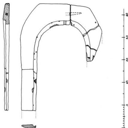
Fig. 4. Fragment af romansk *vinduesramme , udtaget af korets nordmur, 1:10 (s. 2289). Målt og tegnet af Torben Hjelm 1980. - Fragment of window frame, removed from north wall of chancel, 1:10.
