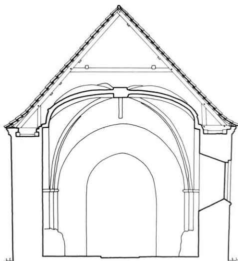
Fig. 3. Snit gennem skib 1:150. Målt af Jens Hougård og Jørgen Viemose 1970, tegnet af Marianne Nielsen 1983. - Section through nave 1:150.
