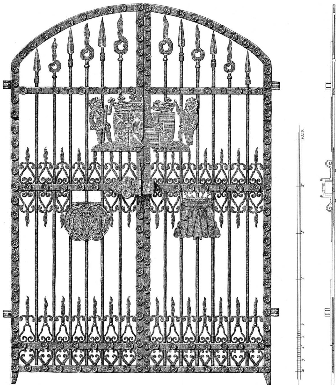
Fig. 36. Smedejernsgitter 1708, til tidligere begravelseskapel for familien Gyldenkrone til Vilhelmsborg (s. 2330). Opmåling 1905 af Anton Frederiksen og K.T.Seest, for Foreningen af 3. decbr. 1892. - Cast-iron lattice door, 1708, to former sepulchral chapel belonging to the Gyldenkrone family of Vilhelmsborg.
