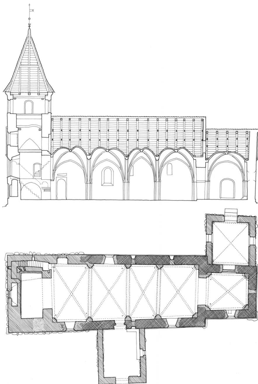
Fig. 8. Plan og længdesnit 1:300. Målt afhenholdsvis C. G. Schultz 1943 og Henrik Jacobsen 1984. Tegnet med enkelte suppleringer af KdeFL 1984. - Plan and longitudinal section 1:300.
