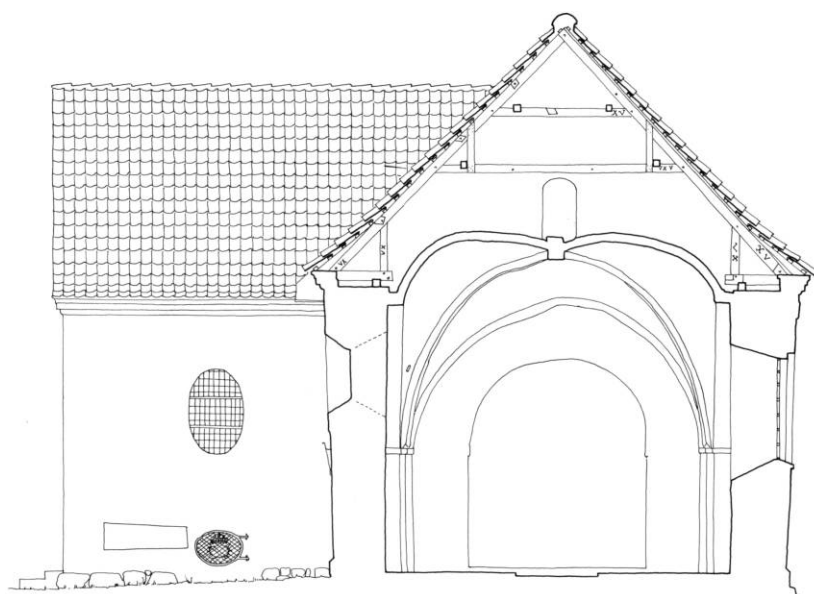
Fig. 9. Tværnsnit gennem skibet, set mod øst med kapellets vestfacade 1:150. Målt af S. G. Petersen 1982, tegnet af KdeFL. - Section through the nave 1:150.
