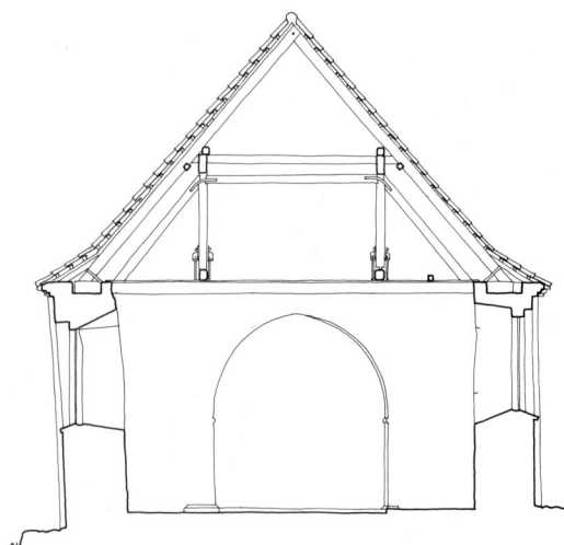
Fig. 5. Tværsnit i skibet 1:150. Målt af Jens Hougaard og Jørgen Viemose 1971, tegnet af KdeFL 1984. – Section through nave 1:150.
