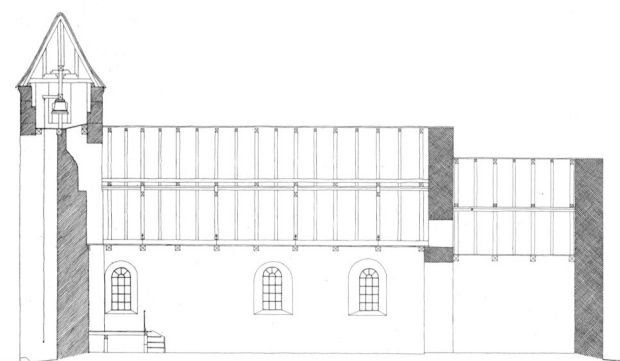
Fig. 4. Sydside, længdesnit og plan 1:300. Henholdsvis målt og tegnet af Svend Pilgaard 1938, målt af Jens Hougaard og Jørgen Viemose 1971, tegnet af KdeFL 1984. – Elevation, section and plan 1:300.
