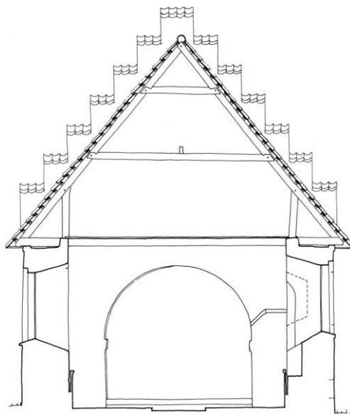
Fig. 7. Snit i skibet, set mod øst 1:150. Målt af Karen Vium Jensen og Preben Skaarup 1972, suppleret og tegnet af KdeFL 1984. - Section 1:150.
