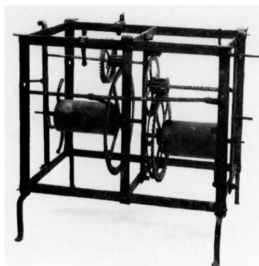
Fig. 25a-b. *Tårnure, skænket mellem 1603 og 1613 af sognepræsten J. Jacobsen (s. 2431). JJF fot. 1984 og opmåling, 1:10, af Søren Andersen 1978. - Tower clock, donated between 1603 and 1613 by the parish priest.
