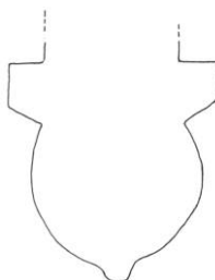
Kysing †kirke. *Profilsten af tegl, 1:5. Privateje. KdeFL 1984 (s. 2440). - Ribbing brick, found beside the ruin.
