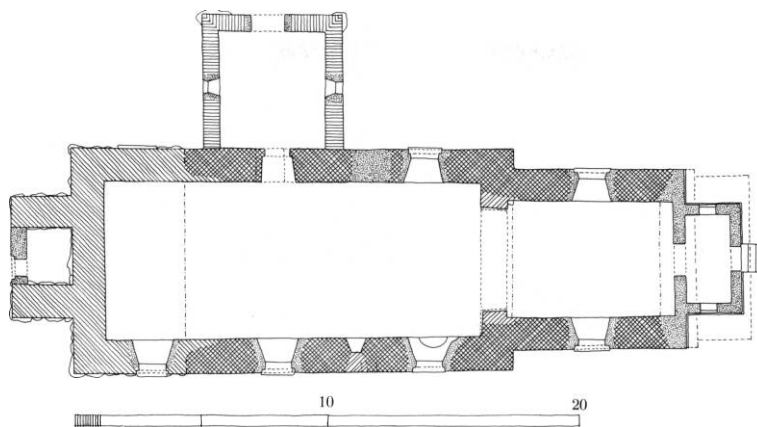
Fig. 6. Grundplan 1:300. Målt af Karen Vium Jensen og Preben Skaarup 1972. Tegnet med iagttagelser ved restaureringen 1981 og med angivelse af den oprindelige korgavl og udstrækningen af det ældre sakristi. KdeFL 1984. - Plan 1:300.
