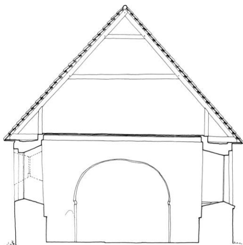
Fig. 3. Snit i skibet, set mod øst, 1:150. Opmålt af Karen Vium Jensen og Preben Skaarup 1972, tegnet af KdeFL 1984. - Section through the nave 1:150.
