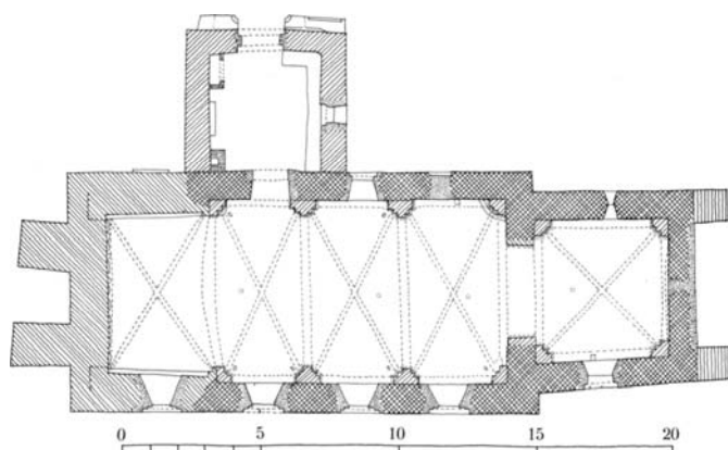
Fig. 2-3. Plan 1:300 og (forneden på siden) tværsnit i skibet, set mod øst 1:150. Opmålt af Jens Hougaard og Jørgen Viemose 1971, tegnet af KdeFL. - Plan of the church and section through the nave, looking east.
