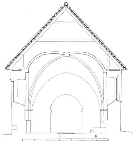
Fig. 3. Tværsnit i skibet, set mod øst 1:150. Opmålt af Jens Hougaard og Jørgen Viemose 1971, tegnet af KdeFL 1985. - Section through the nave.
