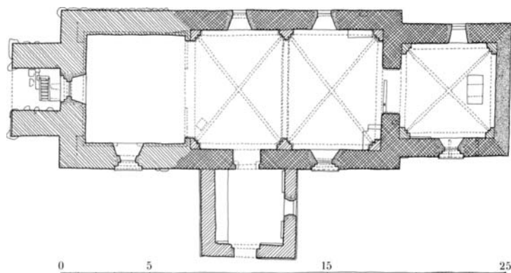
Fig. 2. Grundplan 1:300. Opmålt af Jens Hougaard og Jørgen Viemose 1971, tegnet af KdeFL 1985 med angivelse af de borthuggede anslagsfremspring i sydportalen (s. 2621). - Plan with indication of the cutaway rabbetted projections in the south portal.
