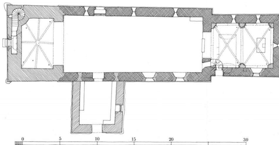
Fig. 4. Grundplan 1:300. Af hensyn til døren er det vestre vindue i korets sydside kun vist med punktering. Målt og tegnet af KdeFL 1985. - Plan .
