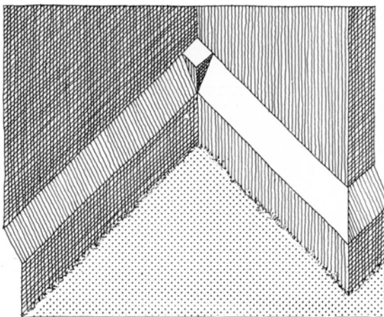
Fig. 6. Skråprojektion af princippet i soklens udformning i hjørnet mellem kor og skib, 1:20 (s. 2651). KdeFL 1985. - The plinth in the corner between chancel and nave.
