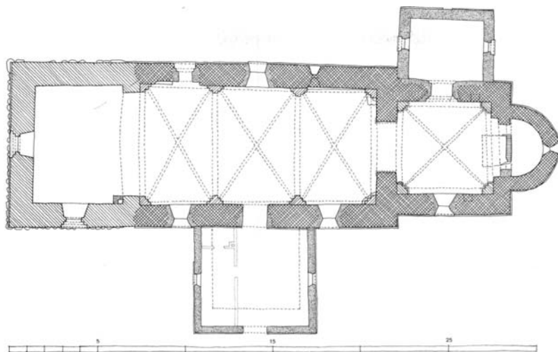
Fig. 6. Grundplan 1:300. Opmålt af Karen Vium Jensen og Preben Skaarup 1972, tegnet 1986 af KdeFL med angivelse af (det indre af) ældre tvåbenhus (punteret) (s. 2721) samt fjernede skillerum i det nuværende (s. 2721). - Plan.
