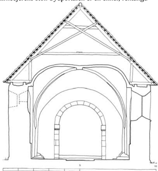
Fig. 7. Tværsnit i skibet set mod øst 1:150. Opmålt af Karen Vium Jensen og Preben Skaarup 1972, tegnet af KdeFL 1986 med udeladelse af tagværksændring 1977. - Section through nave.
