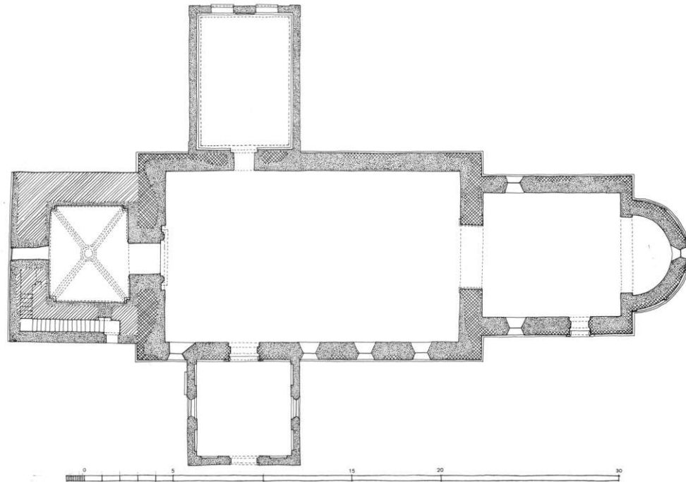
Fig. 4. Plan 1:300. Opmålt af Karen Vium Jensen og Preben Skaarup 1972, tegnet af KdeFL 1986. - Plan.
