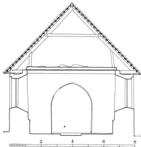
Fig. 4. Tværsnit i skibet, set mod øst 1:150. Opmålt af Karen Vium Jensen og Preben Skaarup 1972, tegnet af KdeFL 1986. - Section through the nave looking east.
