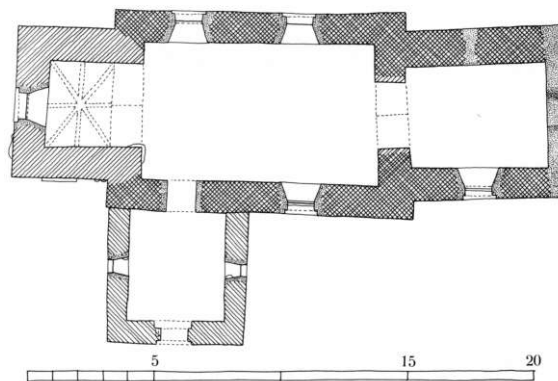
Fig. 6. Grundplan 1:300. Opmålt af Karen Vium Jensen og Preben Skaarup 1972, tegnet af KdeFL 1986. - Plan.
