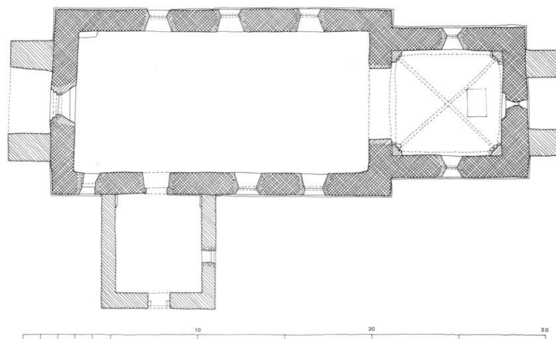
Fig. 2. Plan 1:300. Opmålt 1972 af N. Arndt Andersen, Bue Beck og V. Holten, tegnet af KdeFL 1986. - Plan .
