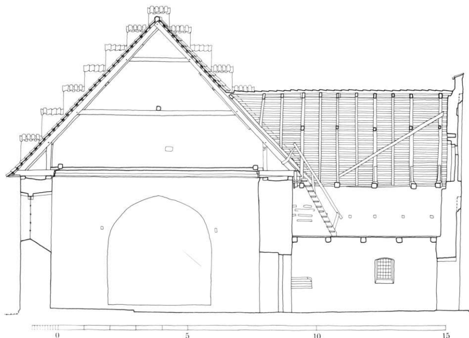
Fig. 3. Snit i skib og våbenhus, set mod øst, 1:150. Opmålt af Niels Arndt Andersen, Bue Beck og Viggo Holten 1972, tegnet af KdeFL 1986. - Section through nave and porch .
