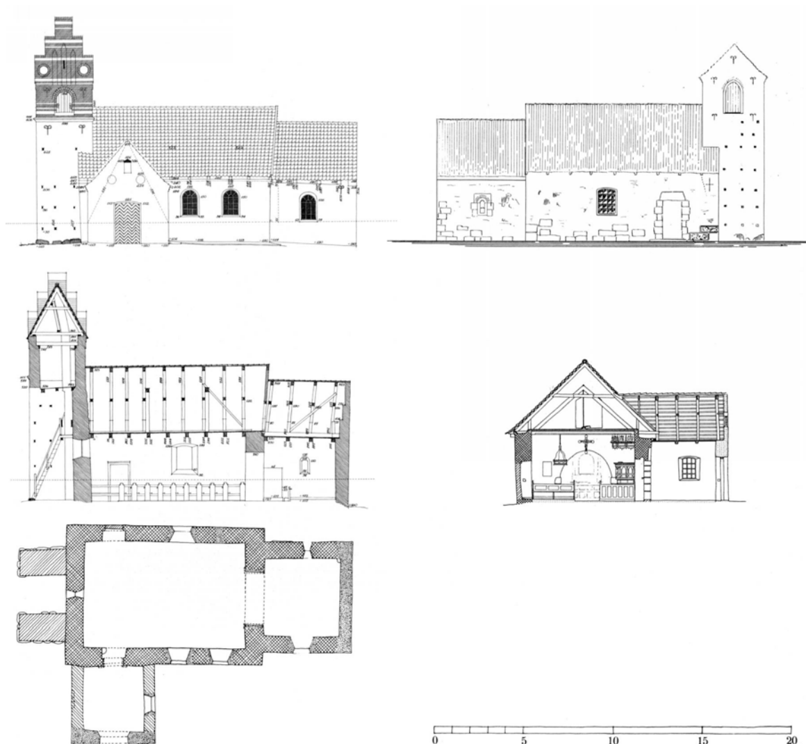
Fig. 4. Opmålinger 1:300. Nordfacade, S. F. Kühnel o. 1885 (Kunstakademiets Bibliotek. Samlingen af Arkitekturtegninger). Sydfacade, Aksel Skov 1951. Tværsnit i skib og våbenhus, Autzen og Jørgensen 1981. Længdesnit, Aksel Skov 1951. Grundplan, KdeFL efter Autzen og Jørgensen 1981. - Elevations, sections and ground-plan.
