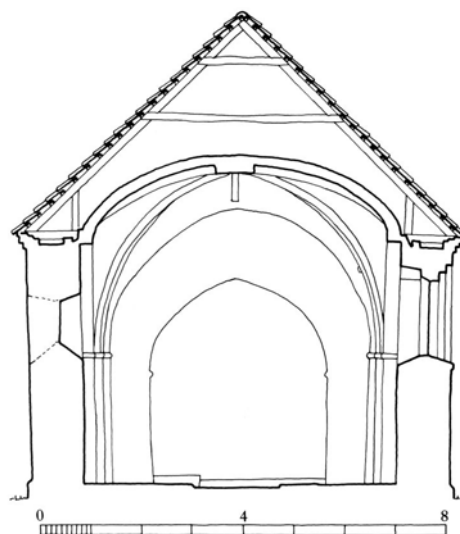
Fig. 5. Tværsnit i skibet, set mod øst 1:150. Tegnet af KdeFL 1988 på grundlag af foreliggende opmålinger. - Cross-section of the nave to the east.
