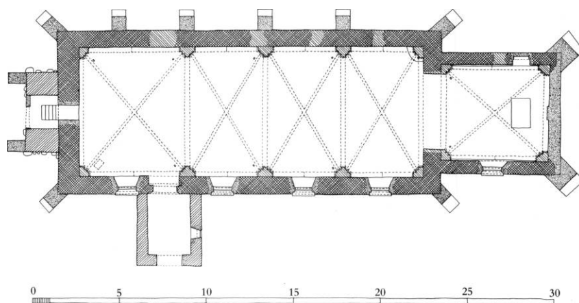
Fig. 3. Grundplan 1:300. Opmålt af Søren Gottfred Petersen 1985, tegnet af KdeFL 1988. - Ground-plan 1:300.
