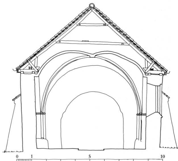
Fig. 4. Tværsnit i skibet set mod øst, 1:150. Opmålt af Søren Gottfred Petersen 1985, tegnet af KdeFL 1988. - Cross-section of the nave to the east.
