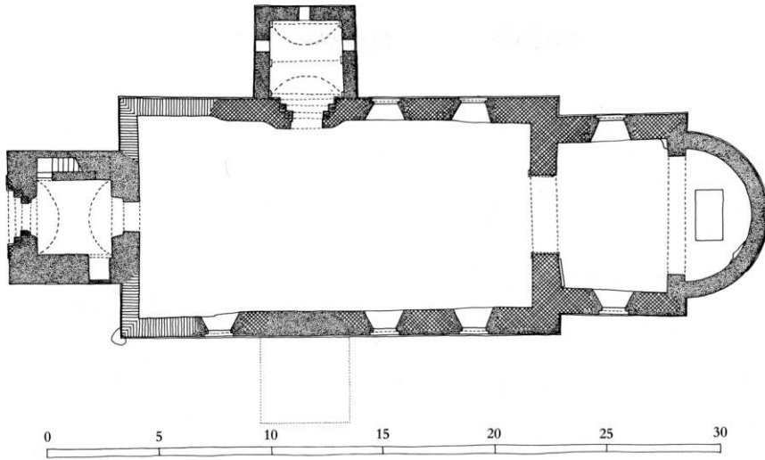
Fig. 3. Grundplan 1:300, opmålt 1983 af Torben Hjelm, tegnet 1989 af KdeFL. En mulig placering og størrelse af et 1792 sløjfet våbenhus på skibets sydside (s. 3278) er angivet med prikket linie. - Ground-plan.
