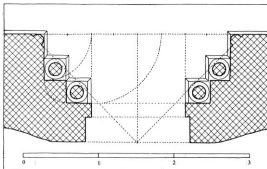
Fig. 9. Nordportal. Forslag til afsætningssystem 1:50. KdeFL 1989 på grundlag af F. Uldalls opmåling. - The north portal. Plan.
