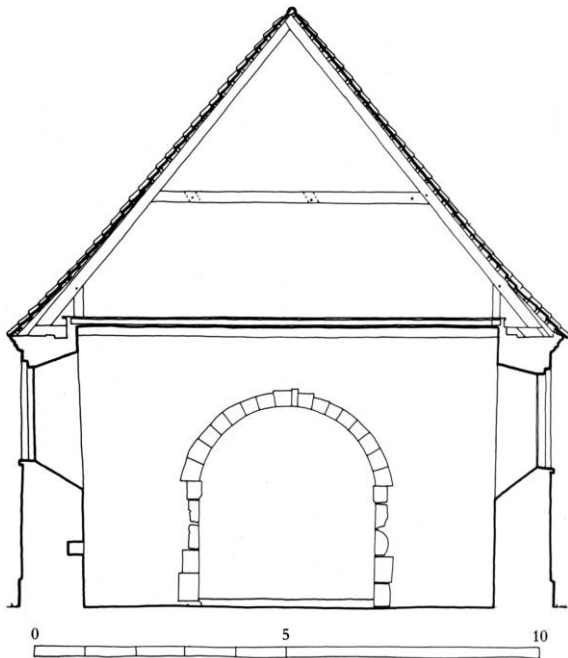
Fig. 4. Tværsnit i skibet, set mod øst 1:150. Målt 1983 af Torben Hjelm, tegnet 1989 af KdeFL. - Cross-section of the nave looking east.
