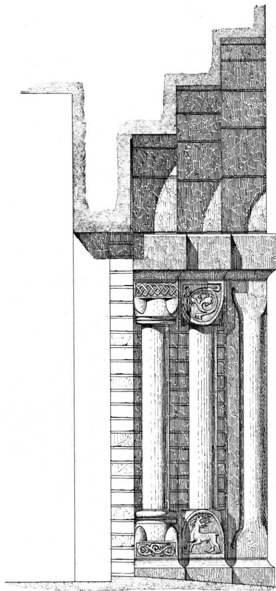
Fig. 5. Sydportalen, der 1792 er placeret på tårnets vestside (s. 3279). Opstalt, plan og snit set mod syd, 1:25. Målt og tegnet 1888 af F. Uldall (s. 3273), der på tegningen har noteret: Tympanon ligger paa Kirkegaarden (s. 3277). - The former south portal, now on the west side of the tower.
