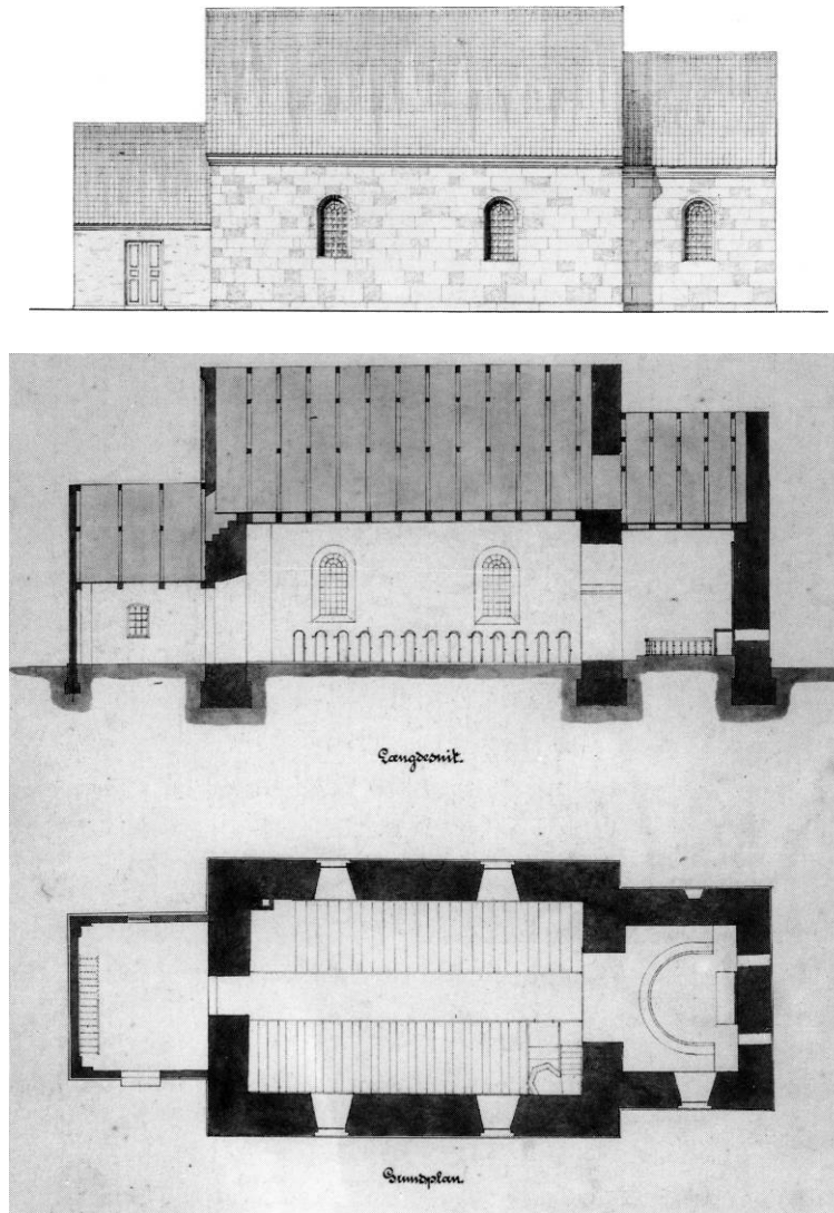
Fig. 6. Opstalt af sydsiden, længdesnit og plan 1:300. Tegnet af Carl Kiilsgaard 1890. Frijsenborg godsarkiv. - Elevation of south side, longitudinal section and plan drawn in 1890.
