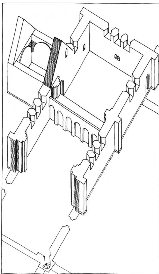
Fig. 7. Første bygningsafsnits første fase (s. 3396). Isometrisk anskueliggørelse 1:300. Indvendige hvælpiller tegnet i deres nuværende skikkelse. †Lektoriets udformning er ukendt (s. 3403). KdeFL 1990. - Proposed reconstruction of the first phase in the building of the church.
