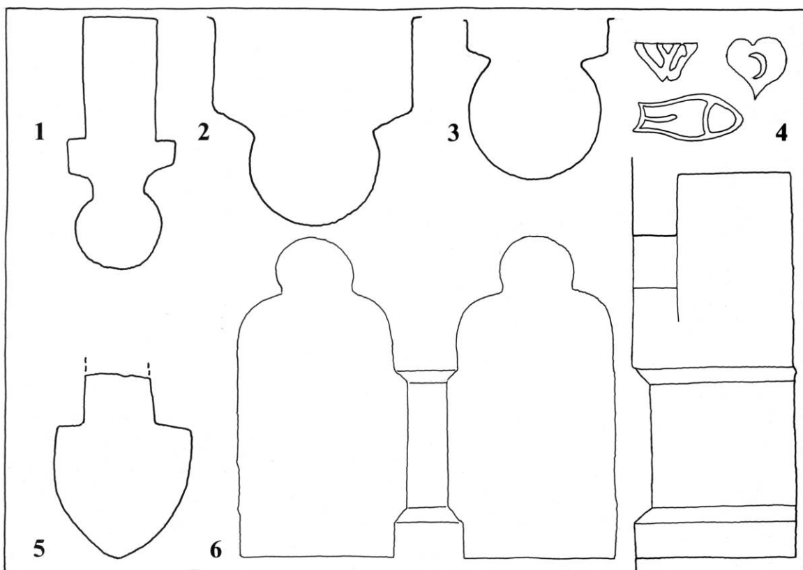
Fig. 16. Enkeltheder tegnet af KdeFL 1990. 1. Ribbesten indmuret i oversiden af hvælvet i kirkens vestligste fag 1:5. 2. Snit i ribbe i kirkens østre afsnit 1:5 (s. 3401). 3. Snit i ribbe i kirkens vestligste fag 1:5 (s. 3405). 4. Stemp-ler fra *vingesten 1:2 (s. 3412). 5. Ribbesten fundet på kirkegården, antagelig fra klosterets vestfløj, 1:5. 6. Niche i kirkens østvæg, opstalt og snit 1:10 (s. 3403). 2, 3 og 6 efter C. Christensen 1925. - Details of the fabric. 1-3 and 5. Cross-sections of ribs. 4. Stamps in *pantiles. 6. Niche in the east wall.
