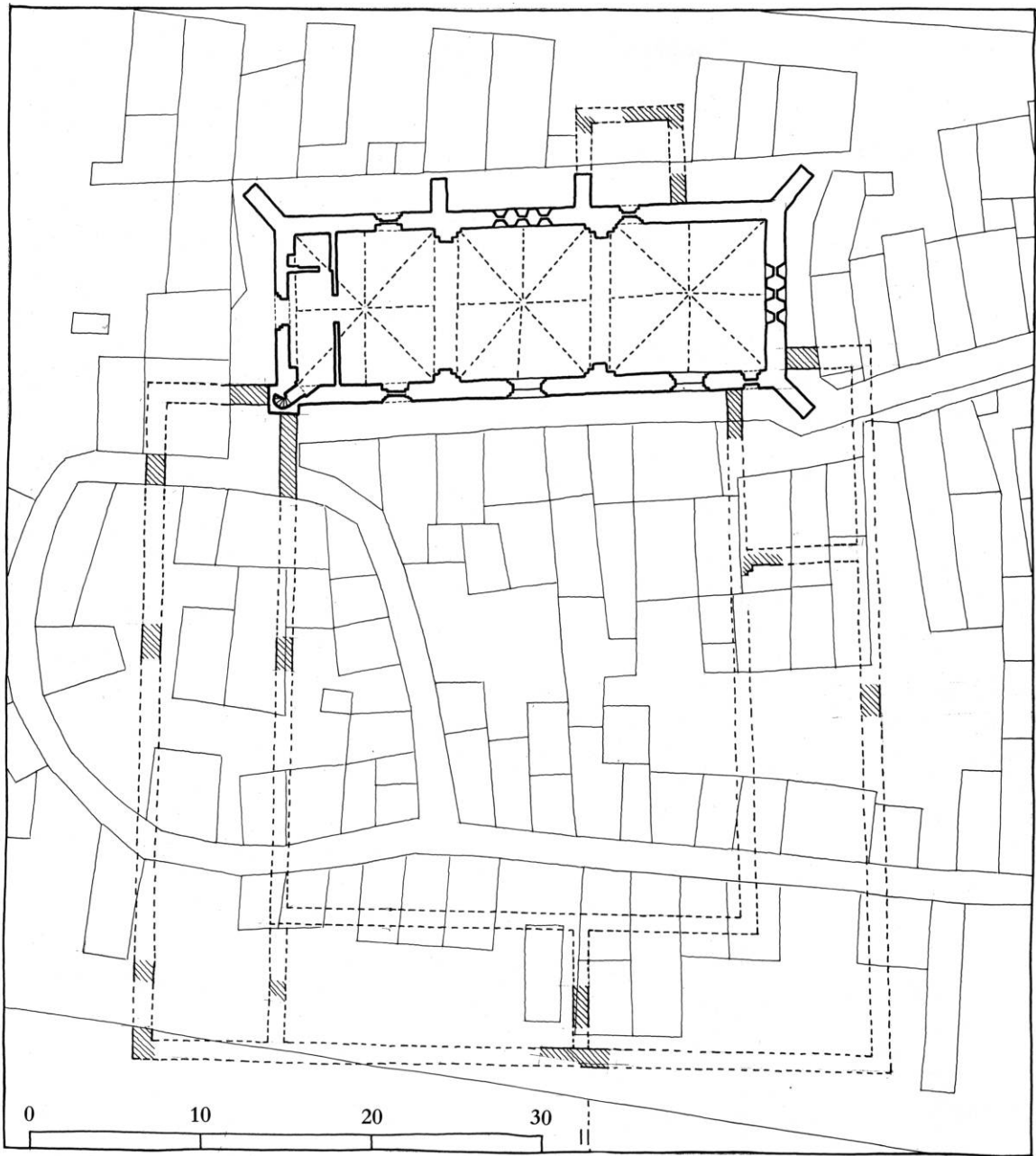
Fig. 3. Tvilum ðkloster. Plan med skematisk angivelse af, hvor der i tidens løb er konstateret bygningslevn, sammentegnet med (udsnit af) kort over gravstedsplaceringer 1912 (LA Vib.), 1:400. KdeFL 1990 på grundlag af C. M. Smidt 1904, B. Meyer 1986 og Middelalderarkæologisk Institut ved Århus Universitet 1990. - Ground-plan of the priory of Tvilum, demolished in the 16th century, with the exception of the church.
