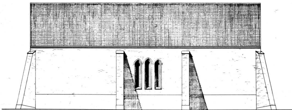
Fig. 5. Nordsiden 1:300. Tegning af Carl Kiilsgaard 1890. Frijsenborg godsarkiv. - Elevation of the north side.
