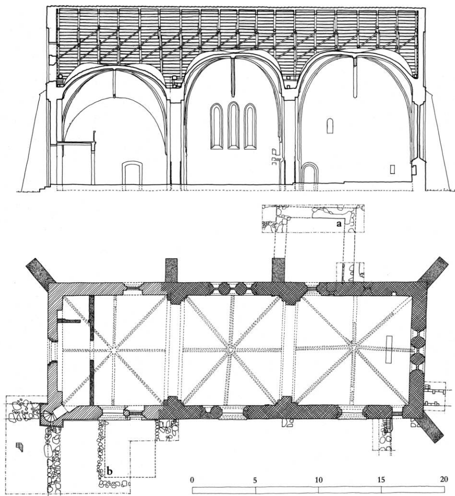
Fig. 6. Længdesnit, efter skitse af B. Meyer 1986, og grundplan 1:300, målt af C. M. Smidt 1904 og C. Christensen 1925, tegnet med suppleringer af KdeFL 1990. Konstaterede fundamentslevn m.v. efter B. Meyer, P. Pentz og Middelalderarkæologisk Institut, Århus Universitet, a. †Sakristi (s. 3403), b. †Våbenhus (s. 3406). Desuden er medtaget konstaterede rester af klosterfløje, jfr. fig. 3. - Longitudinal section and ground-plan. a. †Sacristy, b. †Porch. Also showing remains of the monastery, cf fig. 3.
