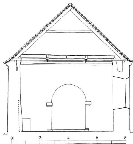
Fig. 2. Tværnsnit i skibet set mod øst 1:150. Opmålt af Cathrine Gerner Hansen 1986, tegnet af KdeFL 1990. - Cross-section of the nave to the east.
