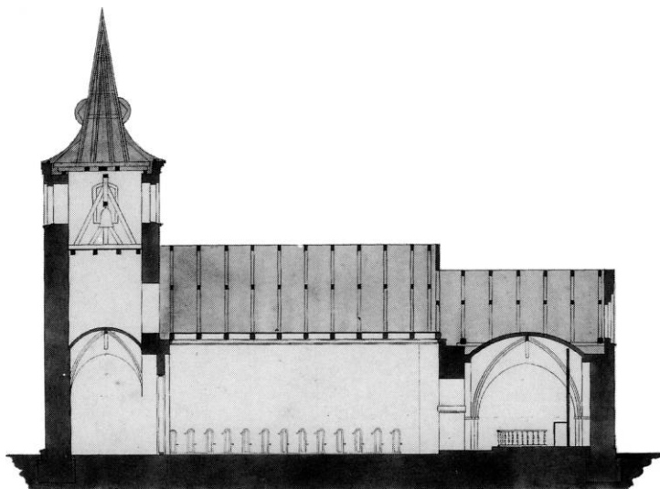
Fig. 3. Længdesnit 1:300. Tegnet af Carl Kiilsgaard 1890, Frijsenborg godsarkiv, Hammel. - Longitudinal section.
