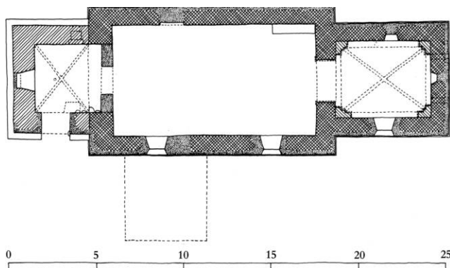
Fig. 4. Grundplan 1:300. Opmålt af Cathrine Gerner Hansen 1986, tegnet af KdeFL 1990. Placering af et eller flere vinduer i skibets nordside kendes ikke. Med punkteret streg er på skibets sydside tegnet omrids af et 1866-67 sløjfet tvåbenhus (s. 3530). - Ground-plan.
