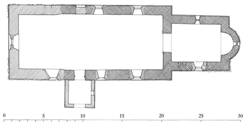
Fig. 9. Grundplan 1:300. Tegnet 1991 af KdeFL på grundlag af Bent Meyer 1972. - Ground-plan.
