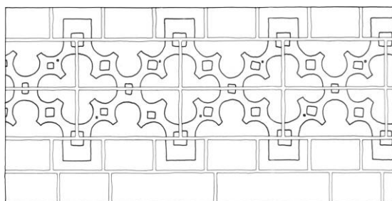
Fig. 13. Skematisk tegning 1:15 af udsnit af frise på kirkens to østre fag. Tegnet af KdeFL 1991 på grundlag af frisen, sten på stedet og sten i NM, jfr. fig. 14 (s. 3722-23 og 2729). - Drawing, 1:15, showing a section of the quatrefoil frieze in the nave's two easterly bays.
