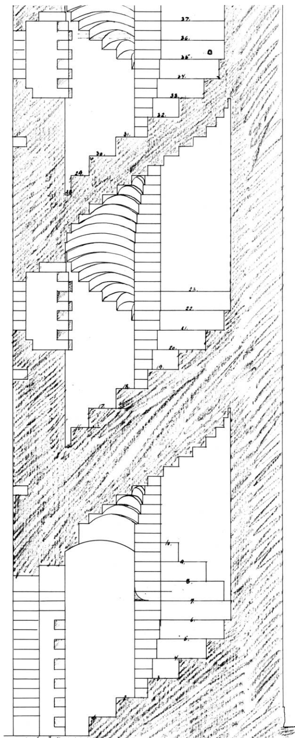
Fig. 16. Udsnit af tårntrappen 1:40 (s. 3732). Hack Kampmanns tegnestuearkiv, Kunstakademiets bibliotek. - Detail, 1:40, of the stairs in the present tower.
