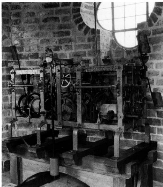
Fig. 44. Tårnuret, udført 1726 af urmager Christian Christensen, Hillerød, til Fredensborg slotskirke, 1913 overført til Rye kirke (s. 3755). NE fot. 1991. - Tower clock, made in 1726 by clockmaker Christian Christensen, Hillerød, for the royal chapel at Fredensborg Palace, transferred in 1913 to Rye church.
