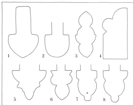
Fig. 12. Formsten 1:10 (s. 2728). Tegnet af KdeFL 1991 efter de eksemplarer, der befinder sig i kirken, undtagen stavværksstenen, der er kopieret efter C. M. Smidt 1910. 1-2. og 5-8. Ribbesten, 3. Stavværkssten og 4. Sten fra vindueslysning (?). - Moulded bricks from the demolished parts of the church.
