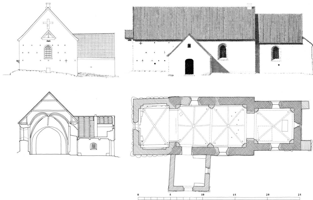
Fig. 4. Opmålinger 1:300. Vestgavl og sydside målt og tegnet af Ida Krøger og Niels Faber 1937-38. Tværnsnit og grundplan målt af Rikke Bøgh, Karsten Juul, Kirsten Knudsen og Klaus Thomassen, Arkitektskolen i Aarhus, 1988, tegnet af KdeFL 1993. - Elevations, sections and ground-plan.
