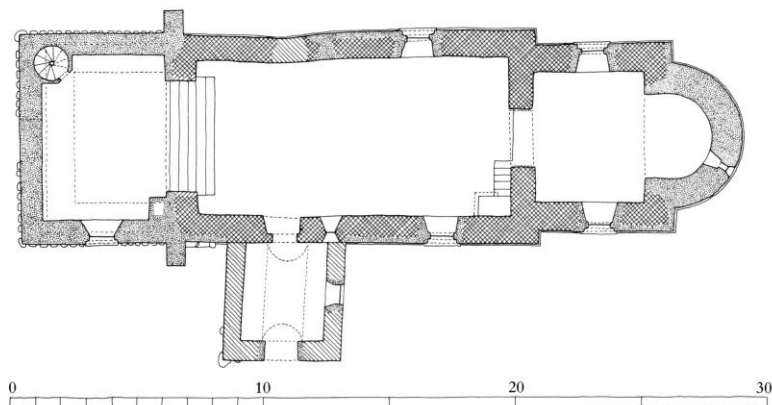
Fig. 4. Grundplan 1:300. Målt af John Bennetzen 1989, tegnet af KdeFL 1993. Med punkteret streg er angivet kontur af \dagger tårn (s. 4080). - Ground-plan .
