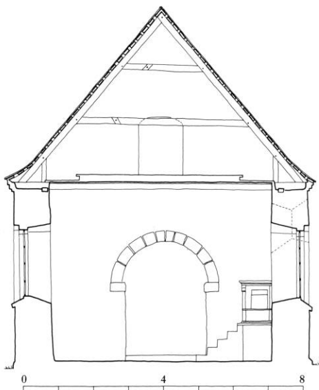
Fig. 5. Tværsnit set mod øst 1:150. Målt af John Bennetzen 1989, tegnet af KdeFL 1993. - Cross-section of the nave looking east .
