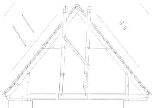
Fig. 26. Et fag af korets tagværk, 1:100 og 1:10. Målt og tegnet af Karen Mundt og Benny Weinreich 1937-38. - Roof truss of the chancel.
