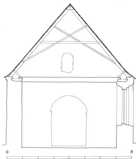
Fig. 5. Tværsnit i skibet, set mod øst 1:150. Målt af Cathrine Gerner og Flemming Aalund 1986, tegnet af KdeFL 1994. - Cross-section of the nave looking east.
