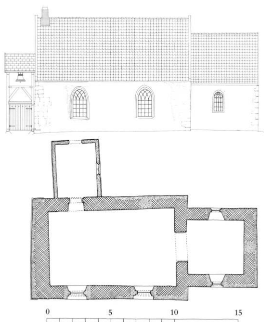
Fig. 4. Sydfacade og grundplan 1:300. Henholdsvis målt og tegnet 1937-38 af Karen Mundt og Benny Weinreich, og målt 1986 af Cathrine Gerner og Flemming Aalund, tegnet af KdeFL 1994. - Elevation of the south facade and ground-plan.
