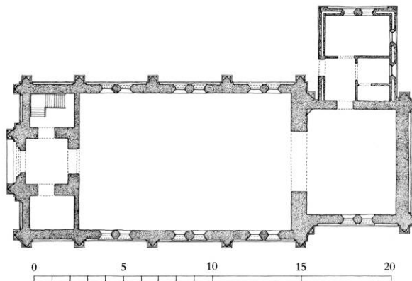
Fig. 3. Grundplan 1:300, justeret og tegnet af KdeFL 1994 efter Hans Vinther 1979 og 1988. - Ground-plan.
