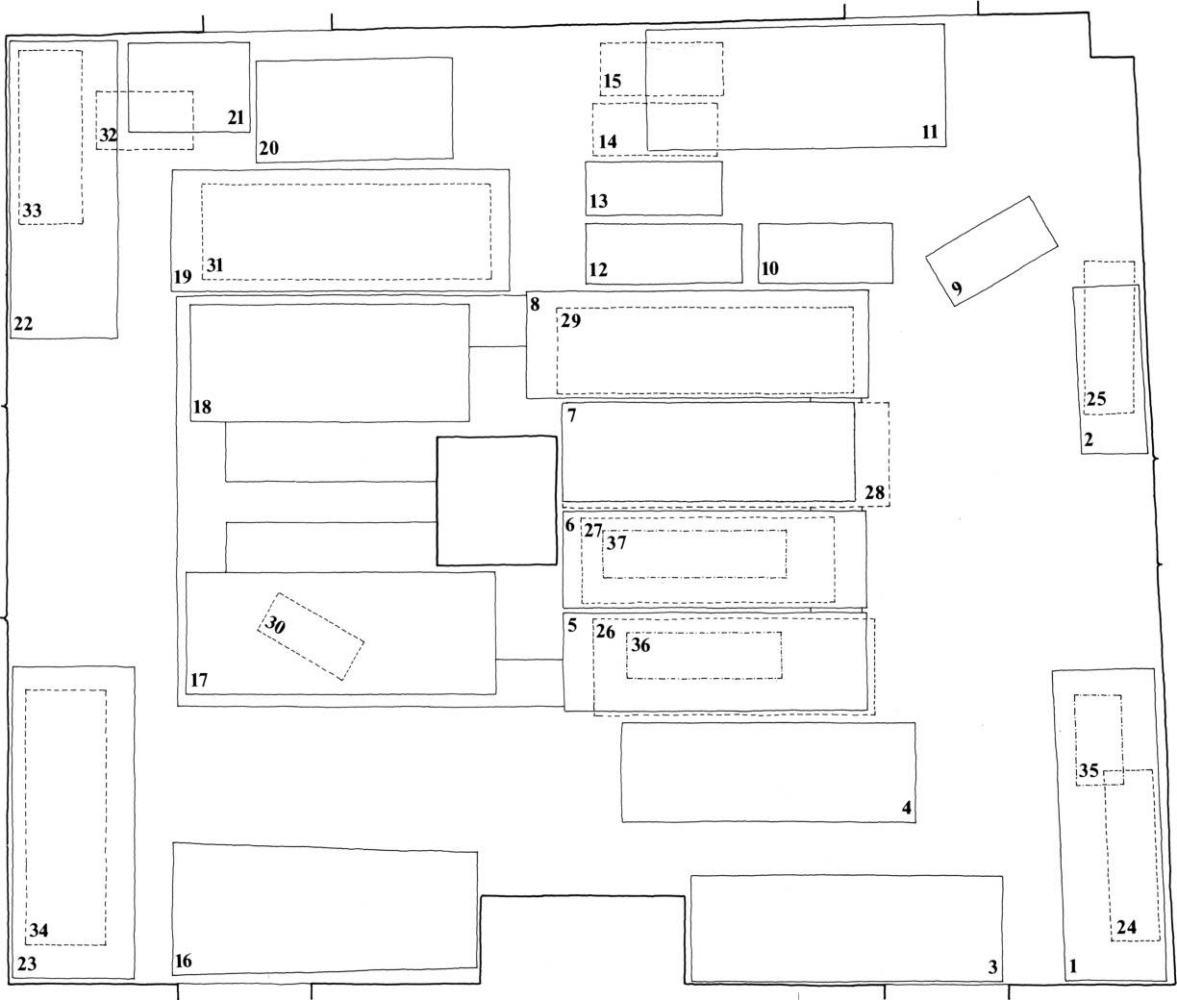
Fig. 53. Principskitse, 1:50, af gravkrypt, jfr. fig. 4, med de nummererede kister. Nederste lag: nr. 1-14 og 16-23, mellemste lag: nr. 15 og 24-34, øverste lag: nr. 35-37. Nord opad. Tegnet af KdeFL 1994. - Sketch plan of the burial crypt, cf. fig. 4, with numbered coffins. Bottom level: nos. 1-14 and 16-23, middle level: nos. 15 and 24-34, top level: 35-37. North above.
