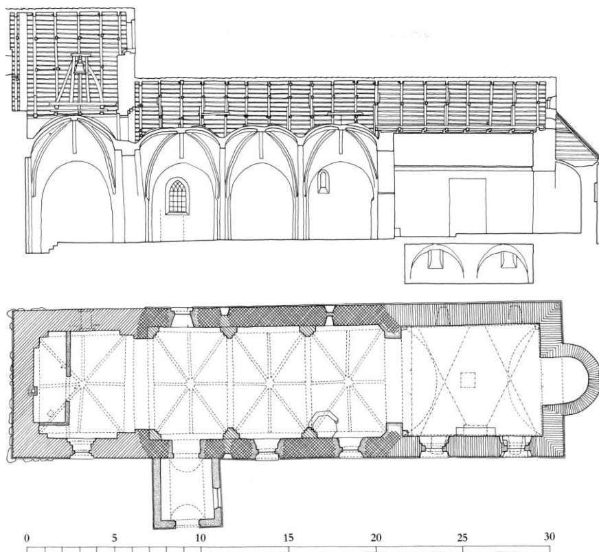
Fig. 4. Længdesnit og grundplan 1:300. Målt af John Bennetzen 1994 og 1992, tegnet og suppleret med skitse af gravrum af KdeFL 1994. - Longitudinal section and ground-plan.
