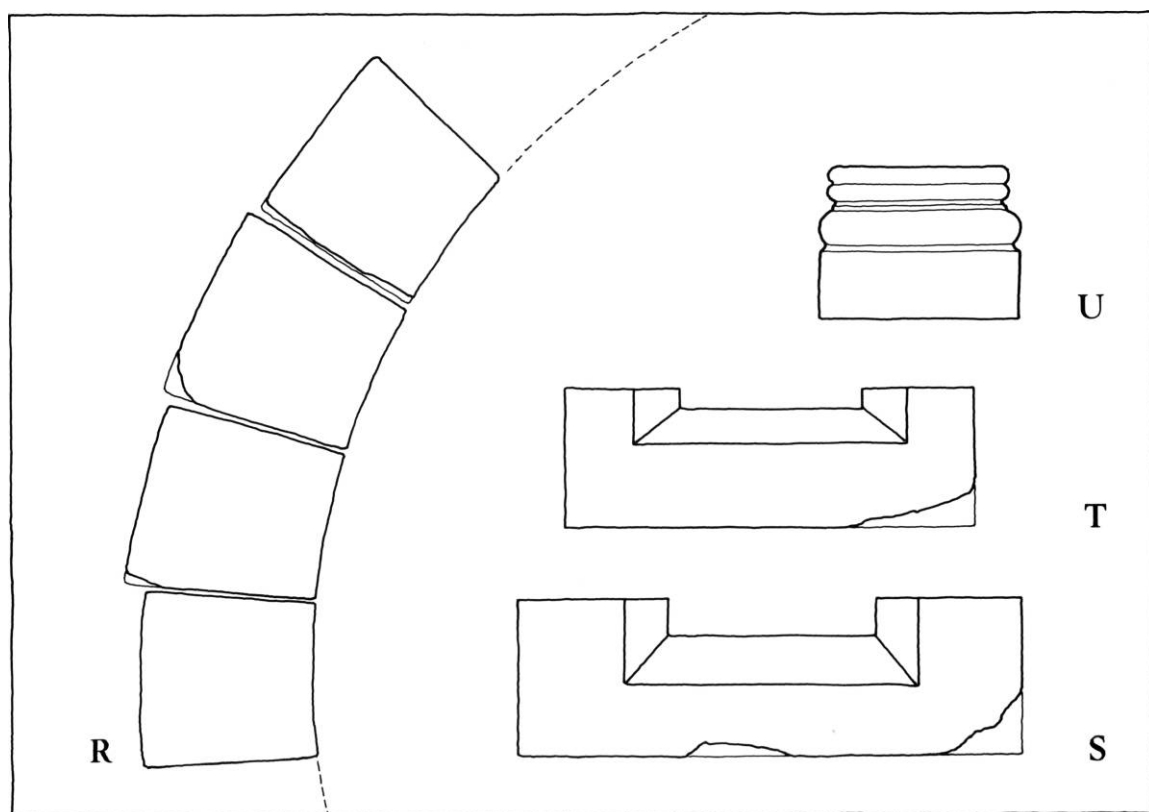
Fig. 7. R-T. 1:20. Særlige kvadre, der sammen med nogle smigsten indgår i tårnets nordre facademur (s. 4259). R. Stiksten. S og T. Sålbenkblokke. U. 1:10. Søjlebase, tidligere indmuret i tårnets vestsideside, nu henlagt i kirken (jfr. fig. 5). KdeFL 1994.- Moulded ashlars and a plinth included in the wall of the tower.
