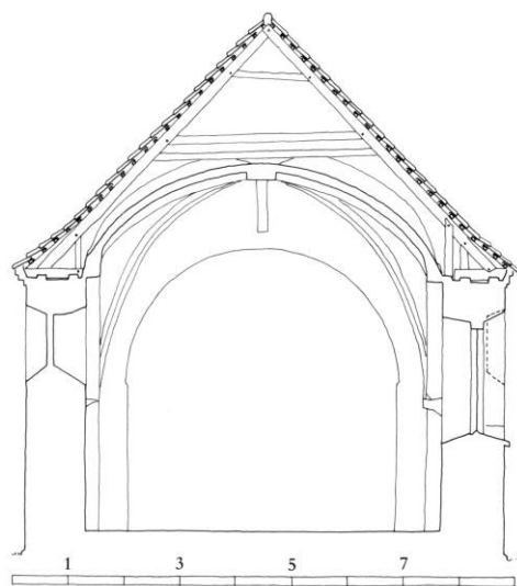
Fig. 6. Tværsnit i skibet set mod øst 1:150. Målt af John Bennetzen 1992, tegnet af KdeFL 1994. - Cross-section of the nave looking east.
