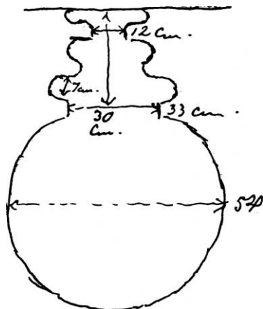
Fig. 70. Tværnsnit af granitplade med forankring i væggen for prædikestolen, jfr. fig. 32 (s. 4276). Skitse af Jørgen Olrik 1913. - Cross-section of granite slab with ties in the wall for anchoring the pulpit, of fig. 32.
