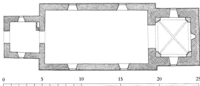
Fig. 4. Plan 1:300. Målt af John Bennetzen 1989, tegnet af KdeFL 1995. - Ground-plan.
