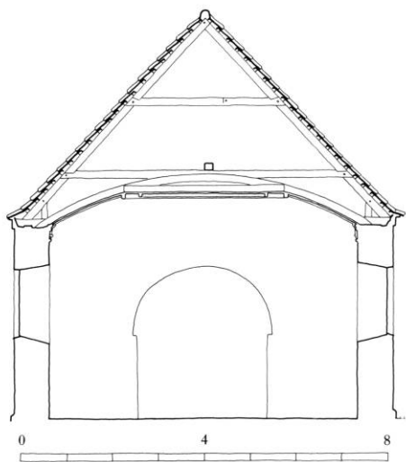
Fig. 3. Tværnsnit i skibet set mod øst. Målt af John Bennetzen 1989, tegnet af KdeFL 1995. - Cross-section of the nave looking east.
