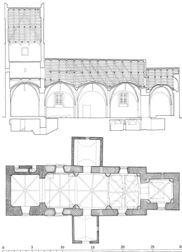
Fig. 7. Længdesnit og plan 1:300. Tegnet med enkelte suppleringer 1995 af KdeFL på grundlag af V. Norn 1934 og Strange Nielsen og Sparre 1970. Under skib og kor er angivet gravrum (s. 4379), på planen tillige kontur af vestafsnittet før ombygning 1934 (s. 4355). - Longitudinal section and ground-plan.
