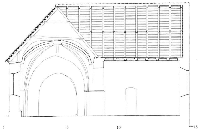
Fig. 10. Tværsnit 1:150. Målt af Johan Bennetsen 1992, tegnet af KdeFL 1995. - Cross section to the east.
