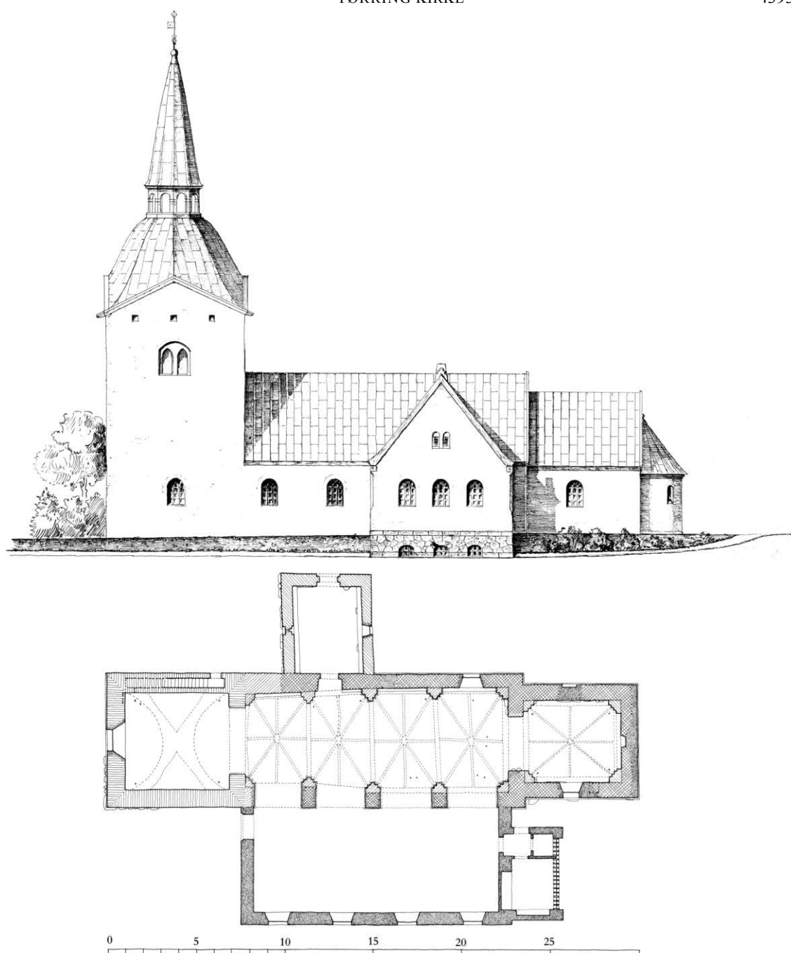
Fig. 4. Ikke benyttet ombygningsforslag af S.F. Kühnel ca. 1910 (s. 4400) og grundplan 1:300 tegnet 1995 af KdeFL på grundlag af bl.a. restaureringsprojekt af Rolf Graae og Richard Aas 1965. - Proposal for rebuilding (not executed), and ground-plan of the present church.
