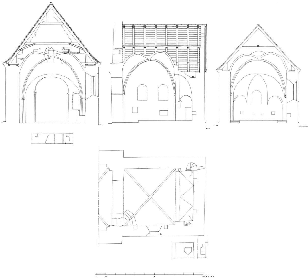
Fig. 6. Skibets østre ende, triumfmur, kor og enkeltheder, snit og plan 1:200. Målt og tegnet af Rolf Graae 1941. - The chancel and the east wall of the nave, sections and ground-plan.
