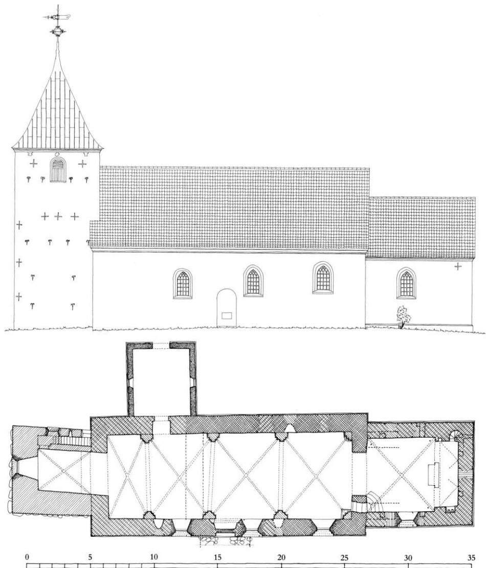
Fig. 5. Sydfacade og plan 1:300. Målt af Rolf Graae 1941 og Vilhelmsen, Marxen og Bech-Jensen 1991, tegnet af henholdsvis Rolf Graae 1941 og KdeFL 1996. - South elevation and ground-plan.
