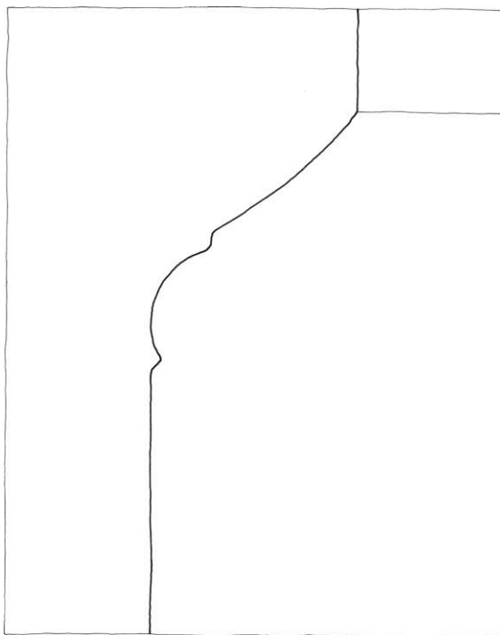
Fig. 12. Skibets sokkel i det sydvestre hjørne (s. 4630), 1:2. KdeFL 1997. - Moulding of the plinth at the south-west corner of the nave .
