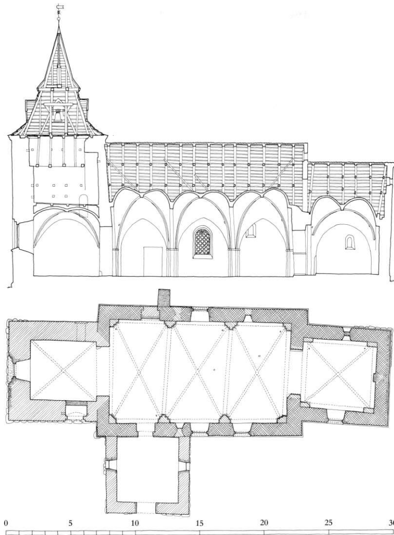
Fig. 5. Længdesnit og grundplan 1:300. Opmålt 1986 afelever fra Byggeteknisk Højskole i Horsens, tegnet 1997 af KdeFL. - Longitudinal section and ground-plan.
