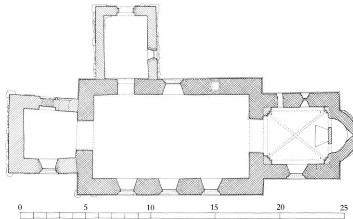
Fig. 4. Grundplan 1:300. Målt af Mads Hjuler og Kurt Lorenzen 1987, tegnet af KdeFL 1997. - Ground-plan
