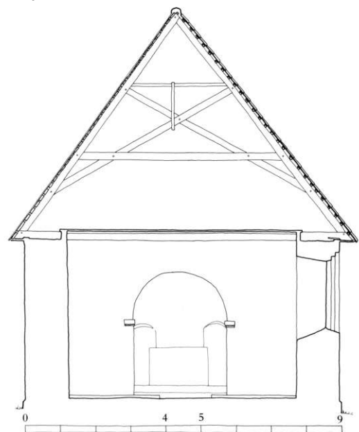
Fig. 5. Tværsnit i skibet set mod øst 1:150. Målt af Mads Hjuler og Kurt Lorenzen 1987, tegnet af KdeFL 1997. - Section of the nave looking east.
