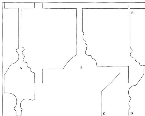
Fig. 5. Profilerede granitblokke 1:10, KdeFL 1997. A. Korbuens vederlagsbånd og sokler (s. 4706). B. Nordportalens kragbånd (s. 4705). C og D. Udvendige sokler (s. 4704). E. *Kragsten fundet 1926 ved Borupgård, nu i Horsens museum (s. 4705). - Moulded granite blocks. A-D from the church, E found in the neighbourhood.
